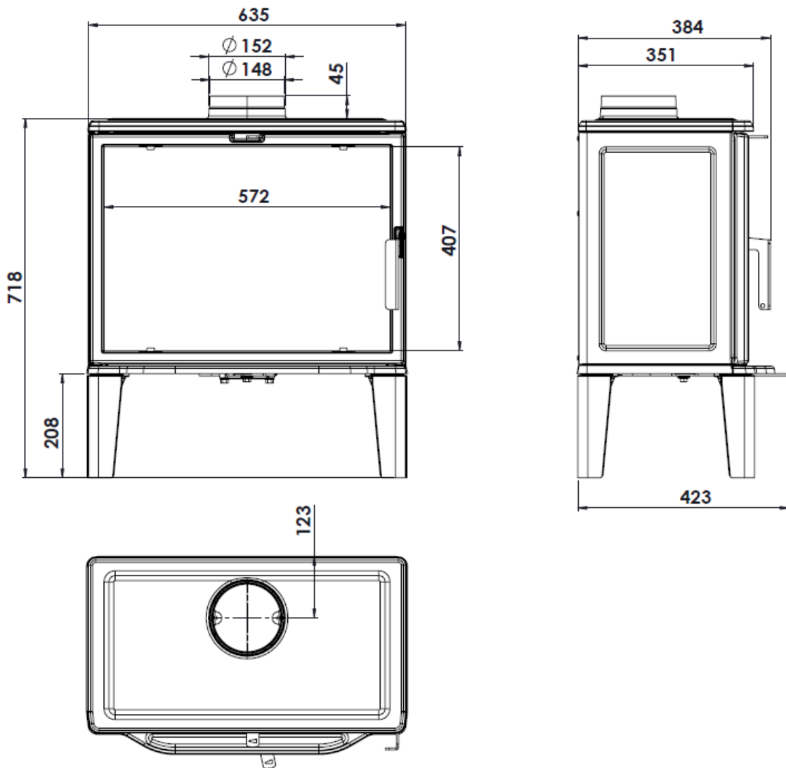
Figure n°1 - Dimensions en mm de l'appareil Biarritz
