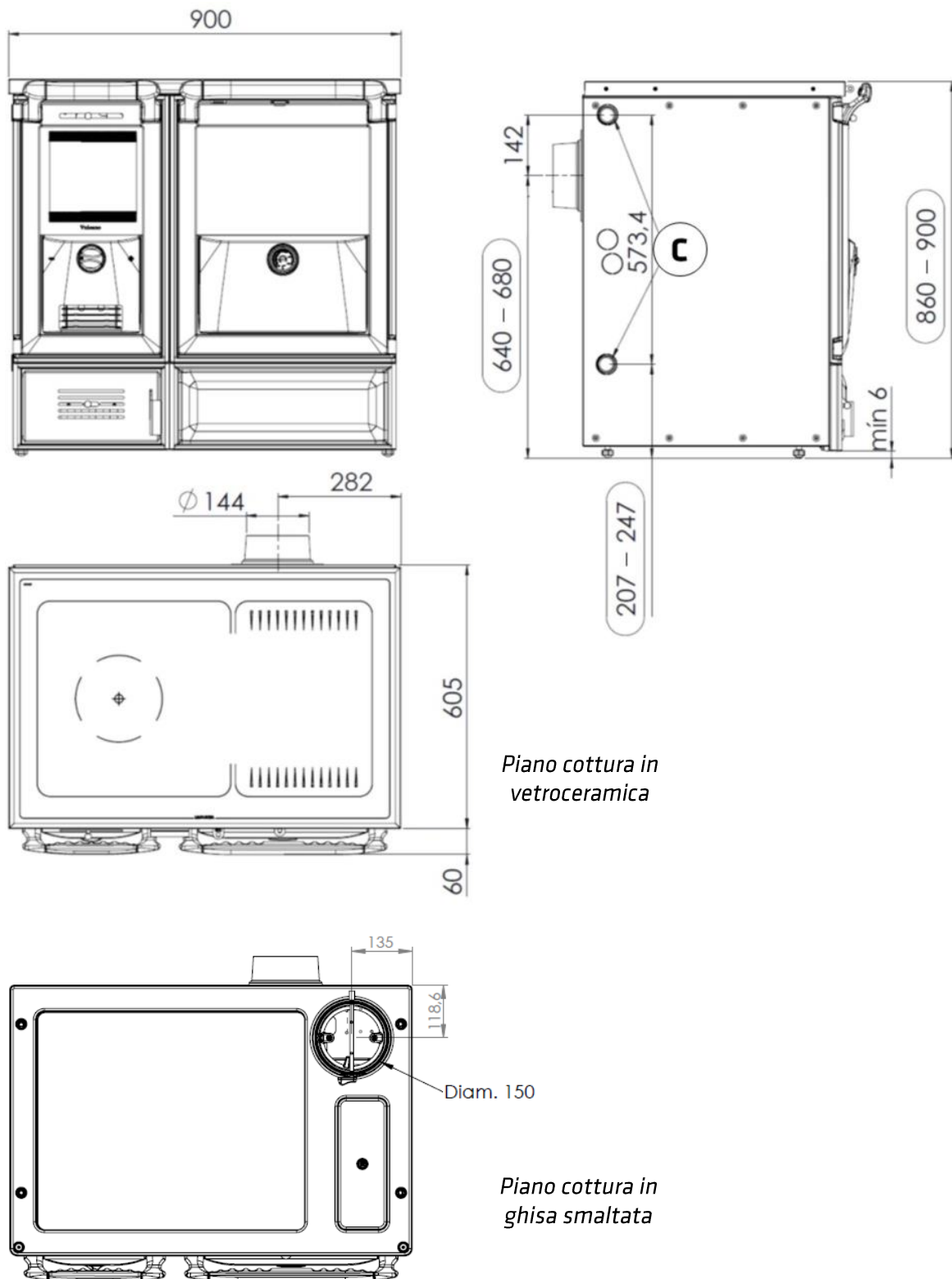
Figura n°3 - Dimensioni in mm dell'apparecchio Vulcano 7T E3
