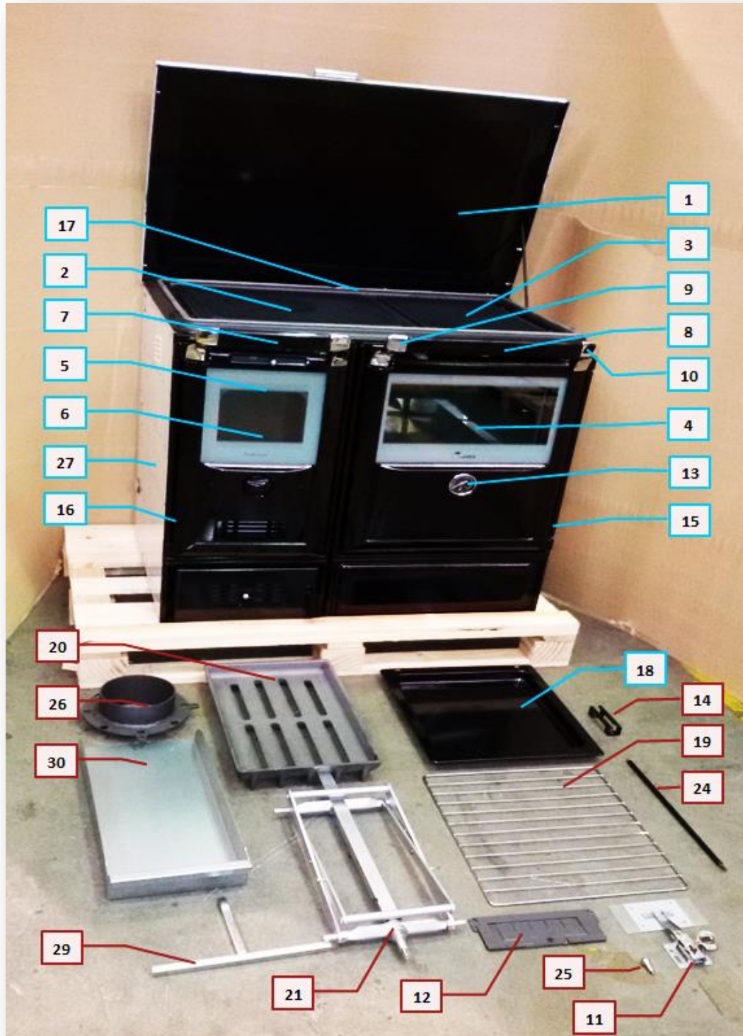
Figure n°35 - Pièces détachées basiques (Vulcano 7TE3)
