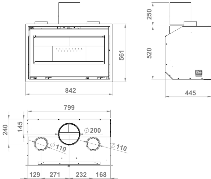
Figure n°2 - Dimensions en mm de l'appareil SILVER 800 PLUS
