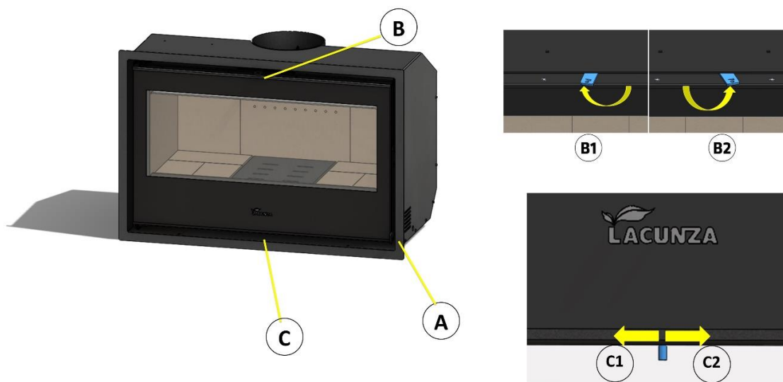
Figure n°6 - Éléments de fonctionnement de l'appareil
