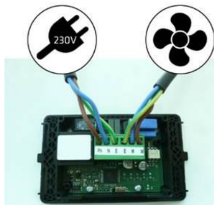
Figure n°1 - Connexions à réaliser au potentiomètre
