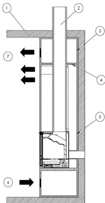
Figure n°5 - Schéma intérieur de la fermeture
