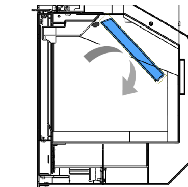
Figure n°10 - Girar y extraer el deflector superior de Acero
