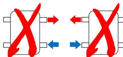
Figure n°11 - Connexions incorrectes (rendement thermique inférieur à l'eau)
