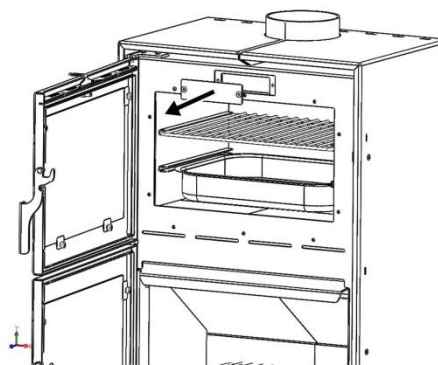
Figure n°15 - Retrait des couvercles d'accès
