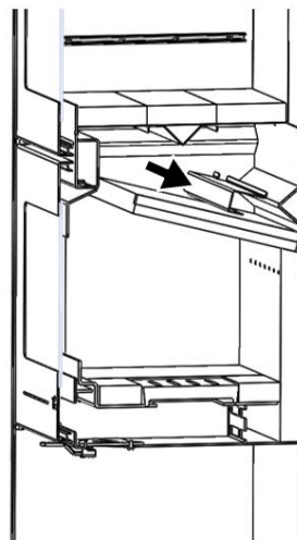
Figure n°13 - Renfort sur les déflecteurs en vermiculite
