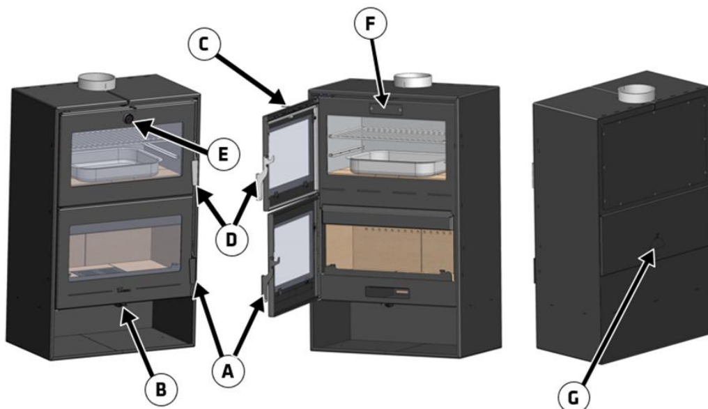
Figure n°7 - Éléments de fonctionnement de l'appareil
