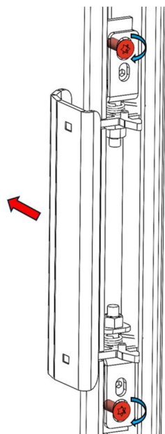
Figure n°6 - ÉTAPE 3 : Serrez les vis pour rattacher le système
