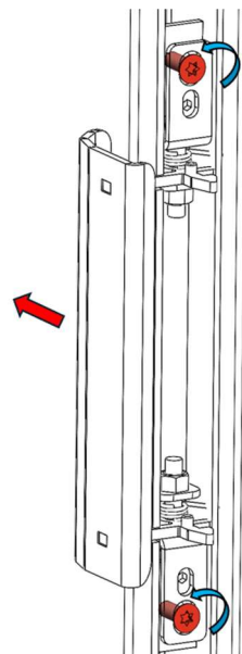
Figure n°4 - ÉTAPE 1 : Desserrez les vis
