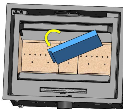
Figure n°23 - Démontage du vermiculite déflecteur plus bas
