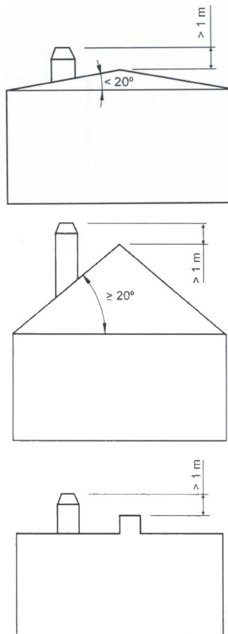
Figure n°18 - Distances depuis le haut du sommet jusqu'au faîtage du toit
