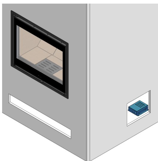
Figure n°17 - Positionnement du boîtier du régulateur devant la bouche d'aération latérale
