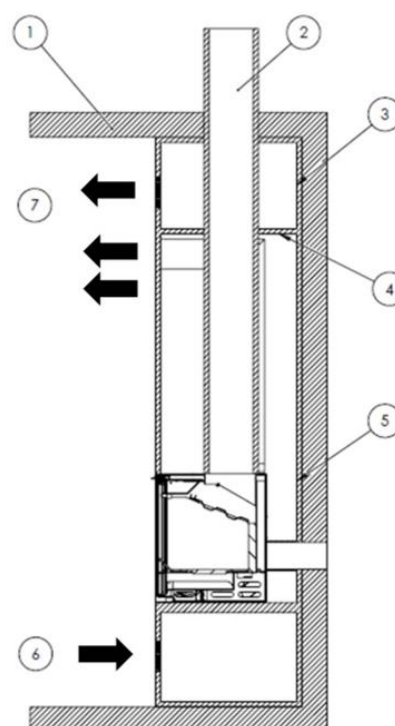
Figure n°5 - Schéma intérieur de la fermeture
