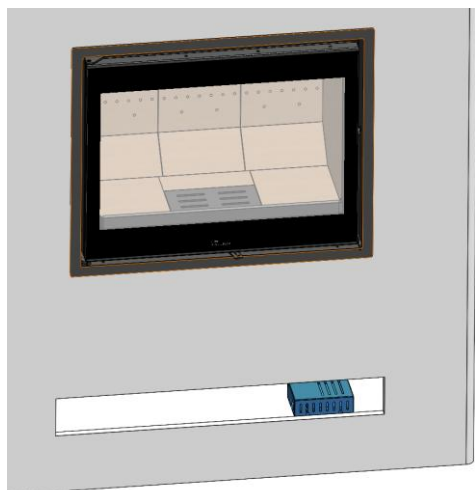
Figure n°16 - Positionnement du boîtier du régulateur devant la bouche d'aération avant
