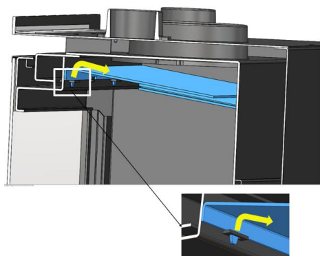
Figure n°24 - Démontage du déflecteur acier
