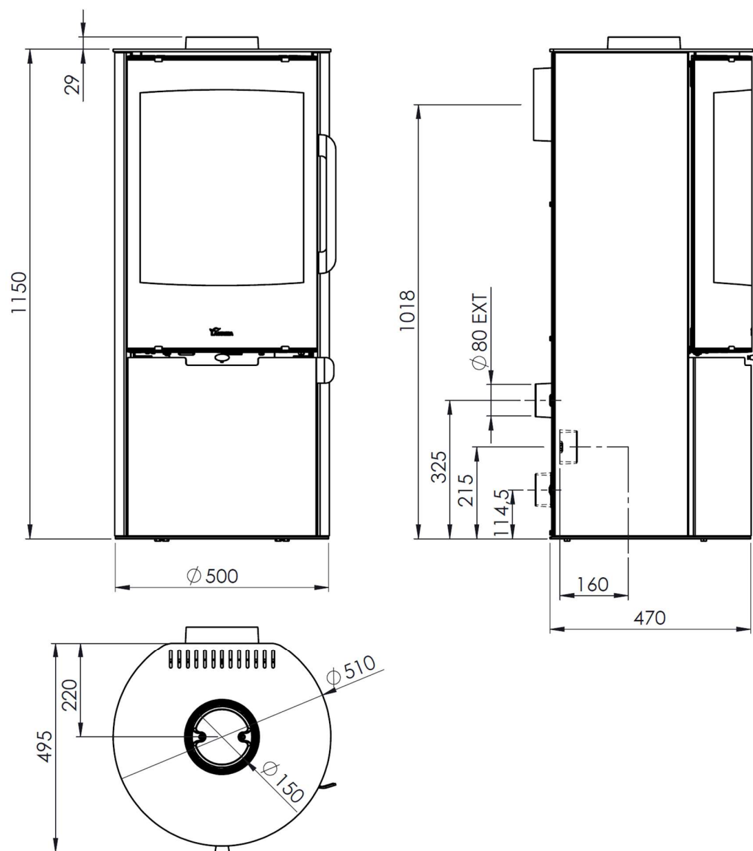
Figure n°1 - Dimensions en mm de l'appareil MAYA et MAYA Vision
