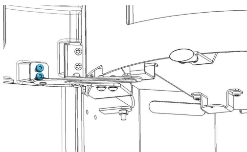
Figure n°26 - Étape 3. Retirer les vis du support de la porte
