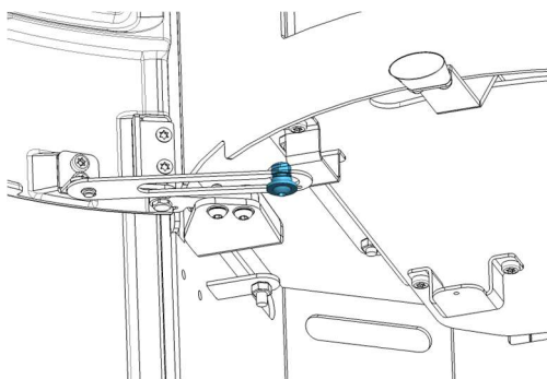
Figure n°25 - Étape 2. Démonter l'arbre
