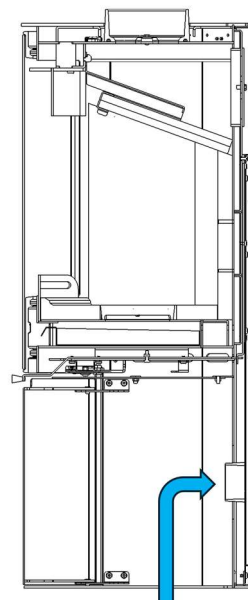
Figure n°9 - OPTION 3 Conduction d'air pour la chambre de combustion
