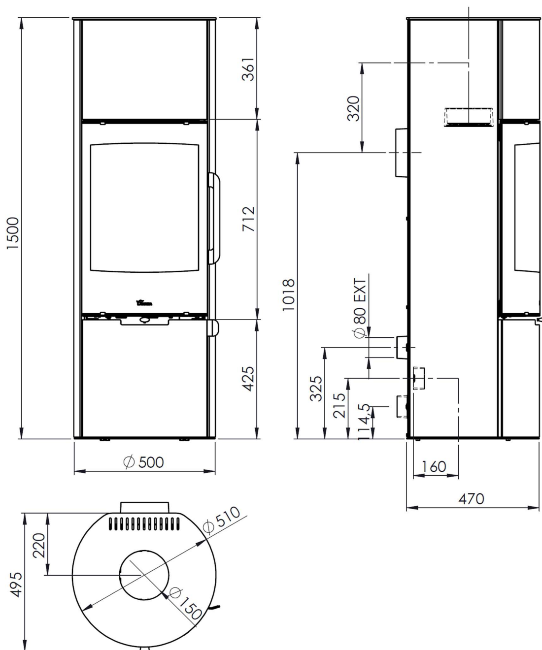
Figure n°2 - Dimensions en mm de l'appareil MAYA ACU et MAYA ACU Vision
