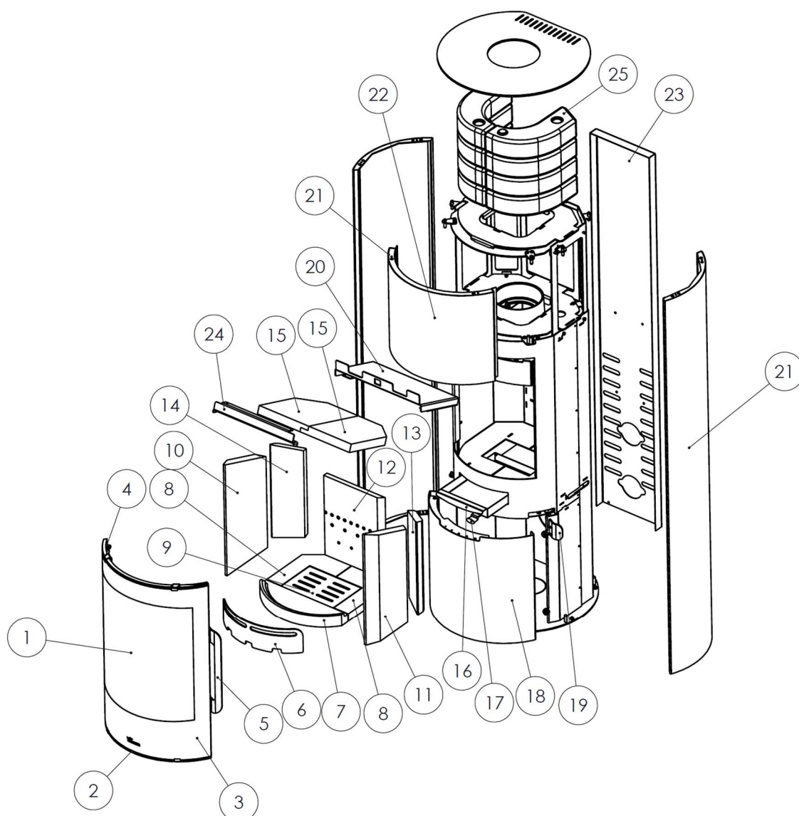
Figure n°4 - Pièces détachées MAYA ACU Visión
