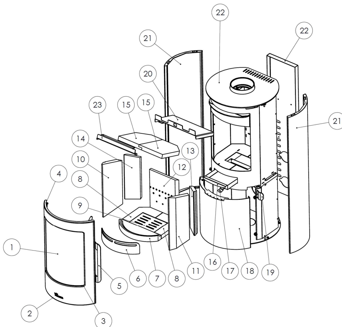
Figure n°1 - Pièces détachées MAYA
