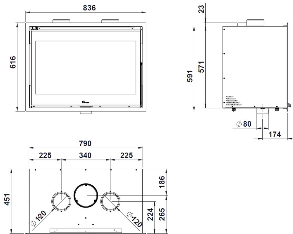
Figure n°2 - Dimensions en mm de l'appareil LOIRE 800
