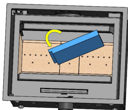
Figure n°24 - Démontage du vermiculite déflecteur plus bas
