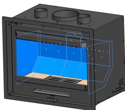
Figure n°24 - Démontage du vermiculite déflecteur plus bas
