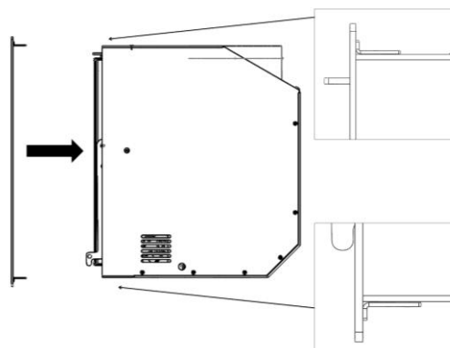
Figure n°15 - Passez l'encadrement par l'intérieur
