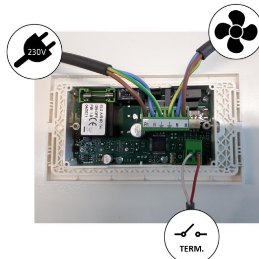
Figure n°1 - Connexions à réaliser au potentiomètre
