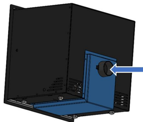
Figure n°7 - Accessoire pour canaliser l'entrée d'air par l'arrière
