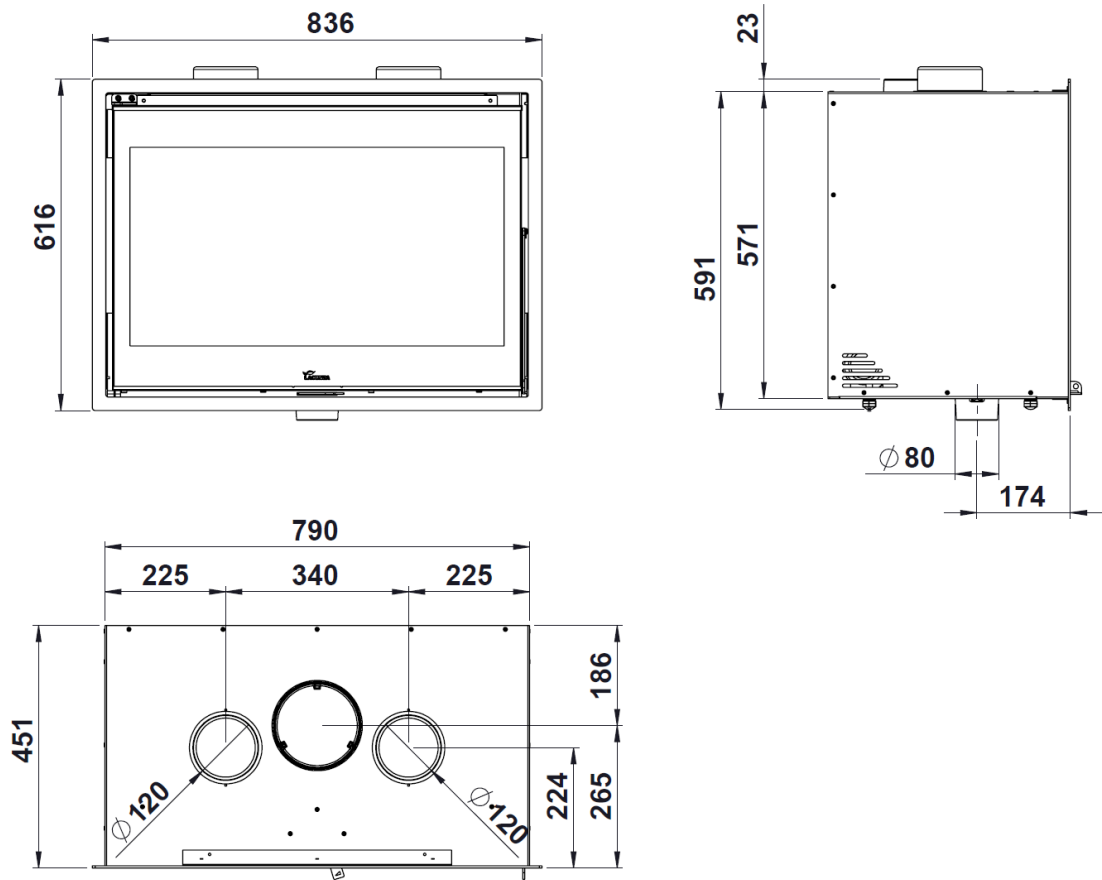
Figure n°2 - Dimensions en mm de l'appareil LOIRE 800
