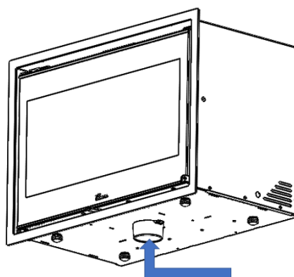
Figure n°6 - Conduction d'air pour la chambre de combustion
