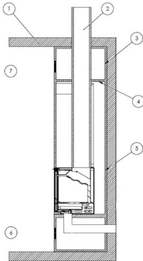
Figure n°4 - Schéma intérieur de la fermeture
