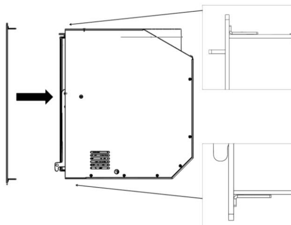
Figure n°12 - Passez l'encadrement par l'intérieur
