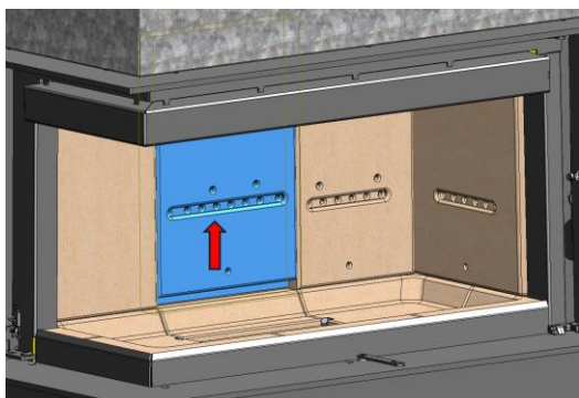
b- Soulever la plaque centrale arrière (5)
