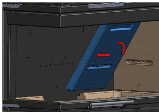
f- Retirer la plaque arrière droite (6) en la déplaçant vers l'intérieur et en la laissant tomber vers l'avant
