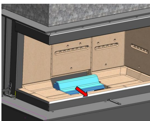
c- Retirez la base centrale arrière (10) en l'avançant.
