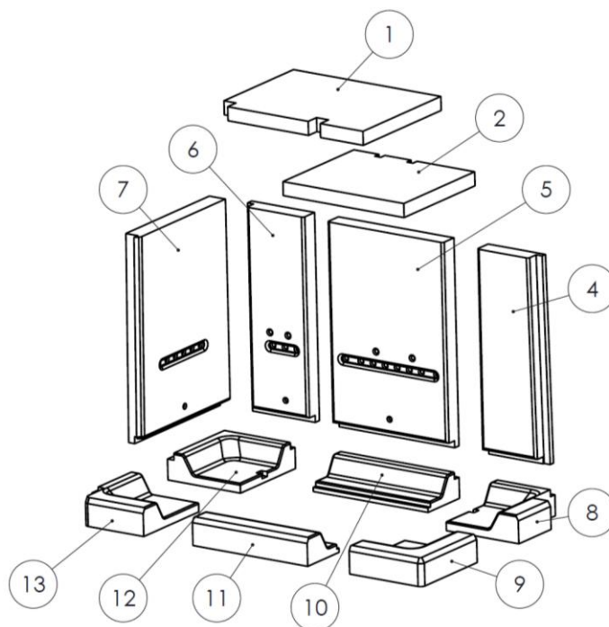
Figure n°52 - Pièces détachées Izaro 80 CLD
