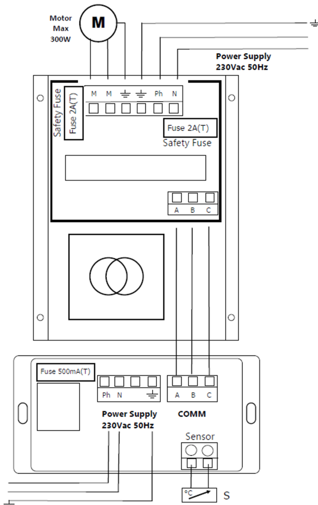
Figure n°20 - Branchements à effectuer dans le contrôleur et le module de puissance de Izaro C/V
