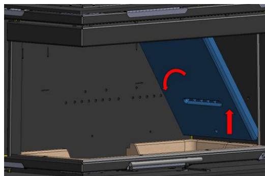
g- Retirez la plaque latérale arrière en la soulevant puis en la laissant retomber vers l'intérieur.
