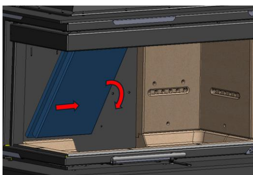
e- Retirez la plaque arrière gauche (4) en la déplaçant vers l'intérieur et en la laissant tomber vers l'avant.
