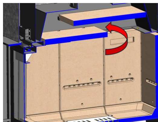
Figure n°31 - Retrait du déflecteur inférieur pour réduire l'enduit IZARO 100 CLI.
