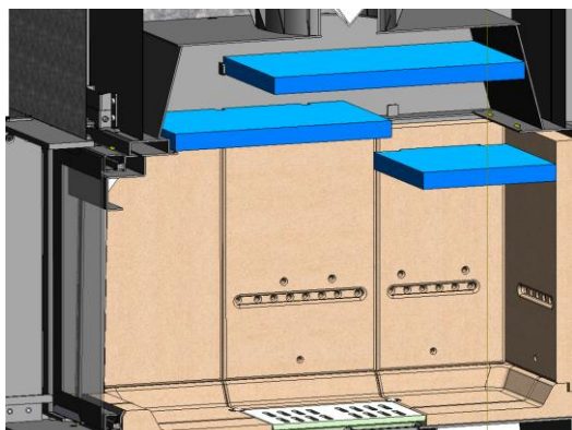
Figure n°34 - Vue de section IZARO 100 CLI avec les déflecteurs placés
