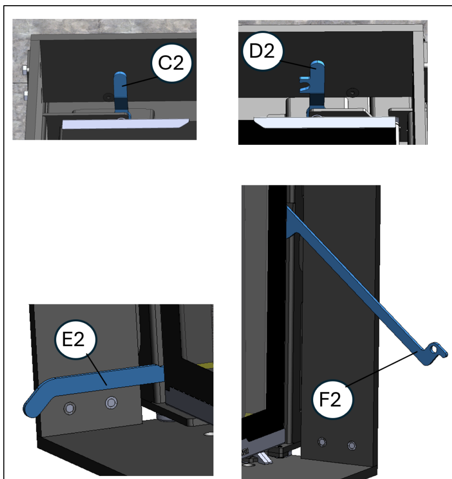
Figure n°29 - Éléments de fonctionnement de l'appareil IZARO 80-100 CLI
