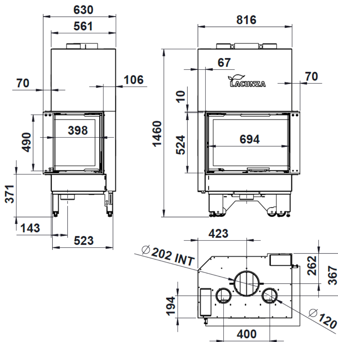
Figure n°3 - Dimensions en mm de l'appareil IZARO 80 CLD
