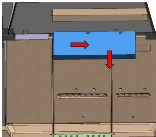
Figure n°36 - Démontage du déflecteur central Izaro 100 CLI
