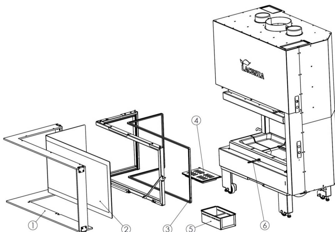
Figure n°48 - Pièces détachées Izaro 80-100 CLI
