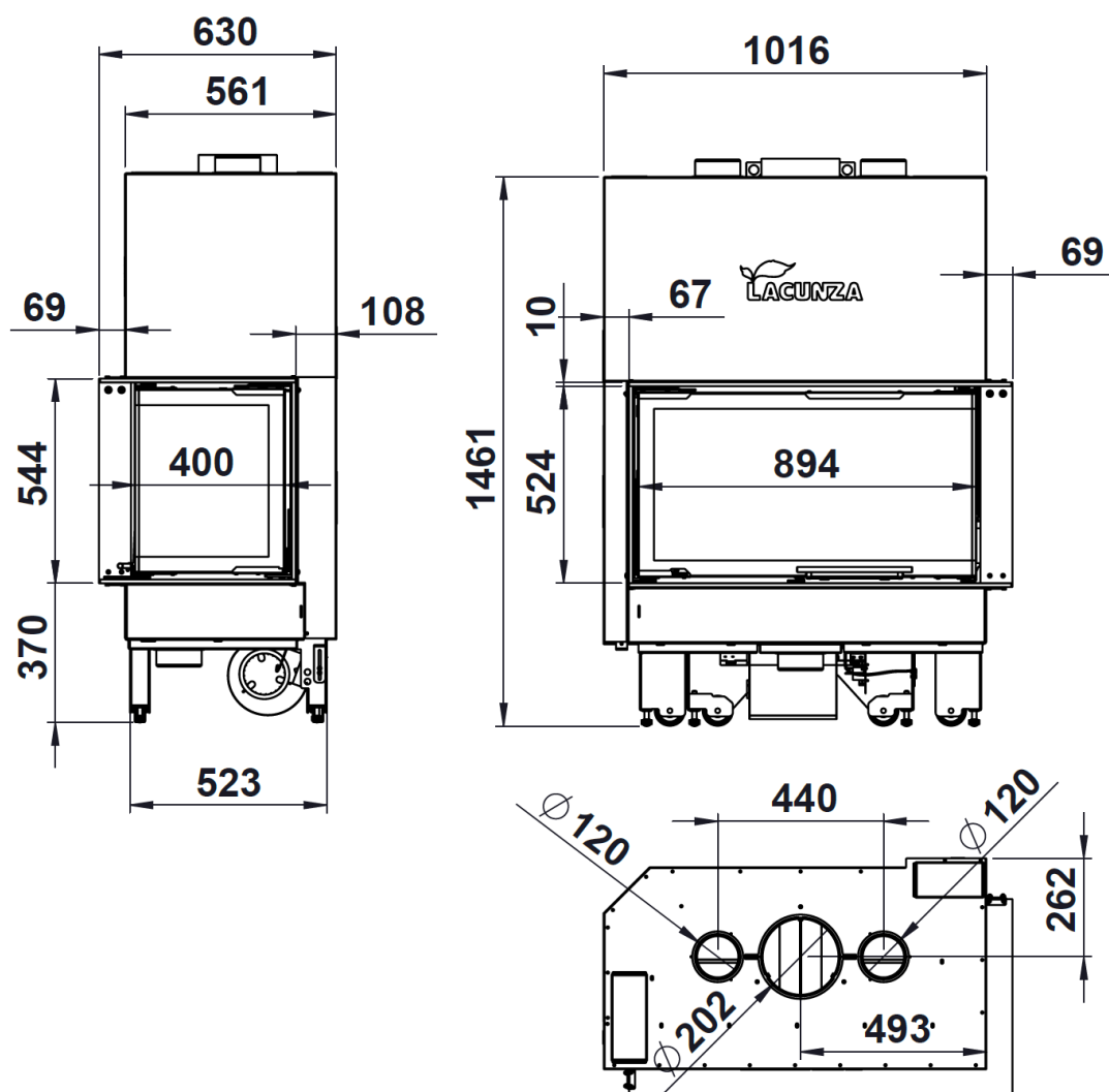
Figure n°4 - Dimensions en mm de l'appareil IZARO 100 CLD
