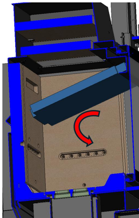
Figure n°35 - Démontage du déflecteur inférieur IZARO 100 CLI
