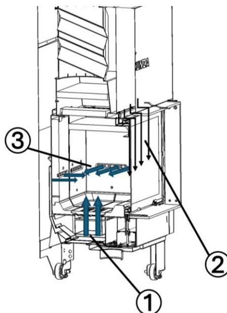
Figure n°32 - Entrées d'air de combustion
