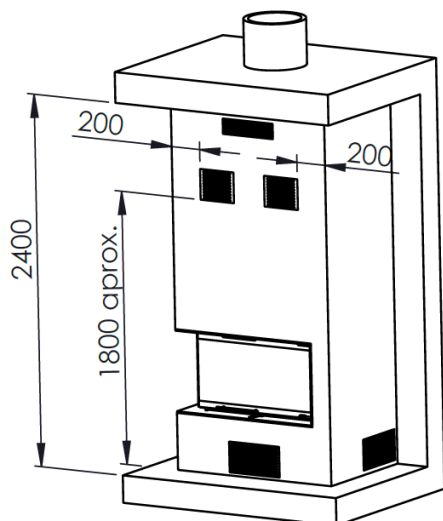
Figure n°10 - Schéma extérieur de la fermeture
