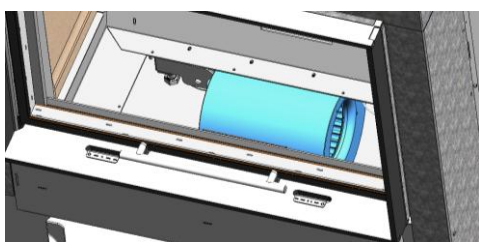
Figure n°46 - Accès à la turbine par l'intérieur de foyer
