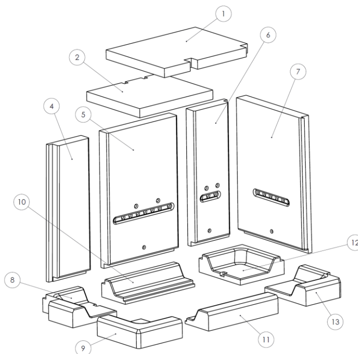
Figure n°49 - Pièces détachées foyer Izaro 80 CLI
