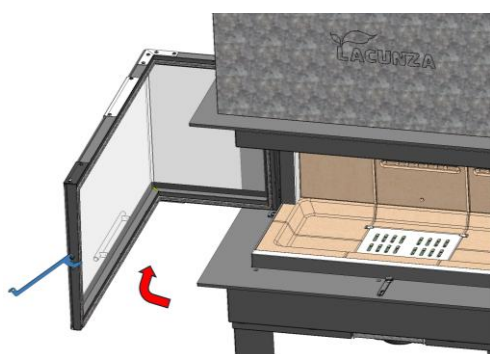
Figure n°43 - Porte ouverte horizontalement
