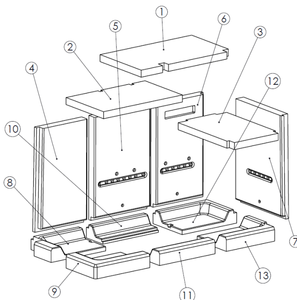
Figure n°50 - Pièces détachées foyer Izaro 100 CLI
