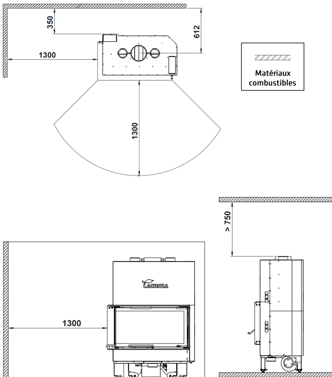
Figure n°5 - Distances de sécurité Izaro 80-100 CLI
