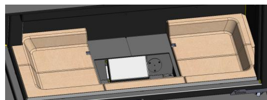
h- Retirer le reste des bases de vermiculite (8), (9), (11), (12), (13).
