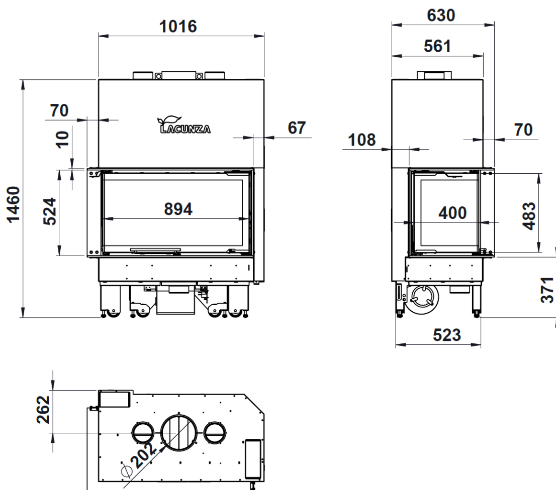
Figure n°2 - Dimensions en mm de l'appareil IZARO 100 CLI
