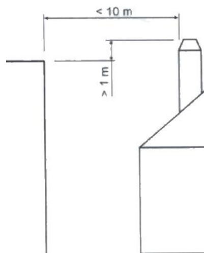
Figure n°26 - Distances entre le sommet et les objets à moins de 10m
