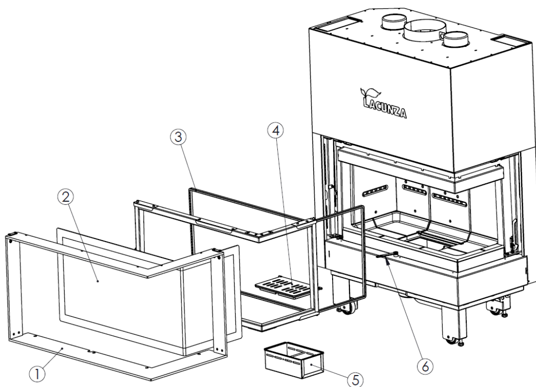
Figure n°51 - Pièces détachées Izaro 80-100 CLD
