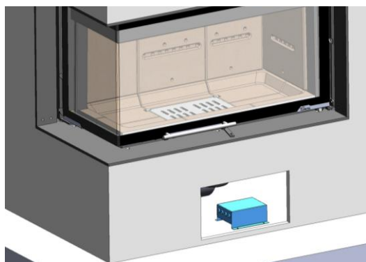
Figure n°22 - Positionnement du module de puissance devant la grille de ventilation avant
