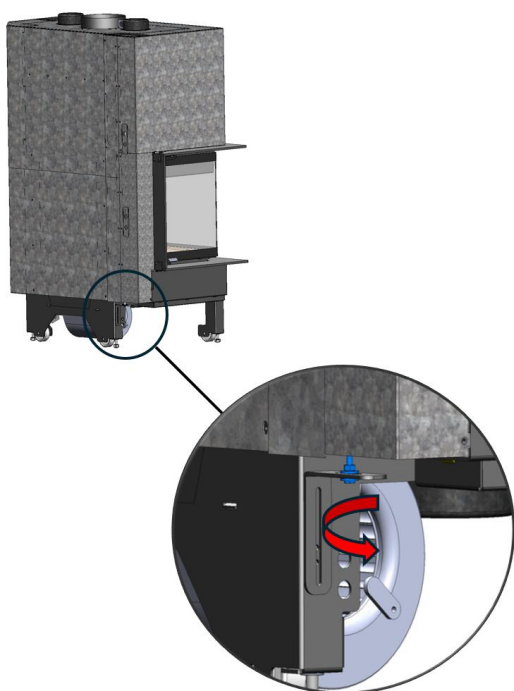
Figure n°7 - Accès pour dévisser les vis de fixation des contrepoids IZARO CLI
