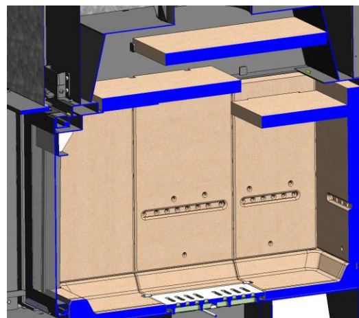
Figure n°30 - Position actuelle de déflecteurs IZARO 100 CLI
