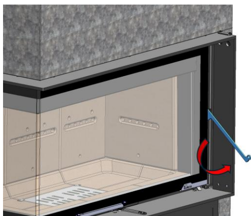
Figure n°42 - Ouvrir la poignée de porte vers l'extérieur.
