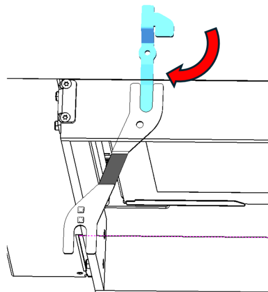
Figure n°41 - Tournez le levier supérieur gauche dans le sens des aiguilles d'une montre de 90°
