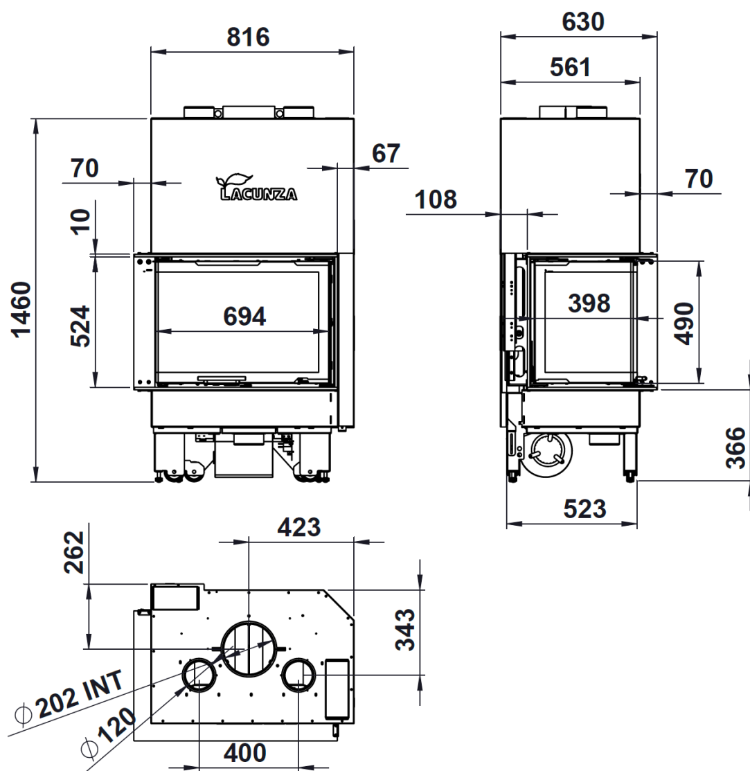
Figure n°1 - Dimensions en mm de l'appareil IZARO 80 CLI
