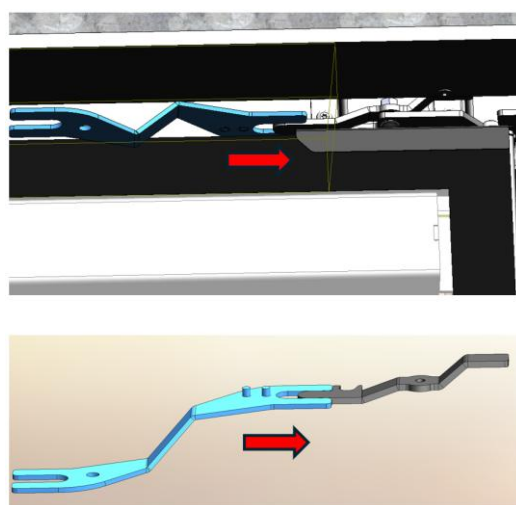
Figure n°39 - Insérer l'outil de manipulation dans le levier rotatif supérieur droit
