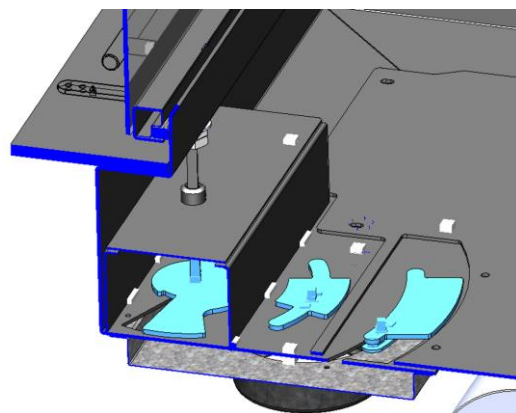
Figure n°47 - Registres amovibles
