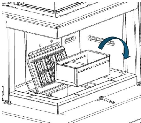
Figure n°33 - Retrait du tiroir cendrier
