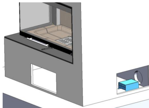
Figure n°23 - Positionnement du module de puissance devant la grille de ventilation latérale
