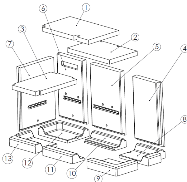
Figure n°53 - Pièces détachées foyer Izaro 100 CLD
