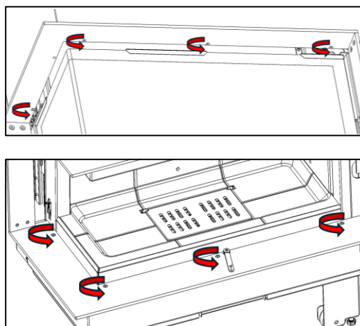
Figure n°17 - Dévissez les 8 vis qui fixent le cadre extérieur, 4 supérieurs et 4 inférieurs
