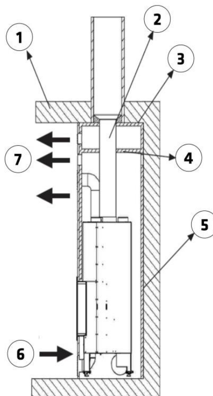
Figure n°9 - Schéma intérieur de la fermeture
