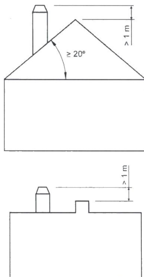
Figure n°25 - Distances depuis le haut du sommet jusqu'au faîtage du toit
