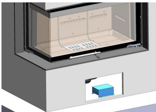
Figure n°20 - Positionnement du module de puissance devant la grille de ventilation avant
