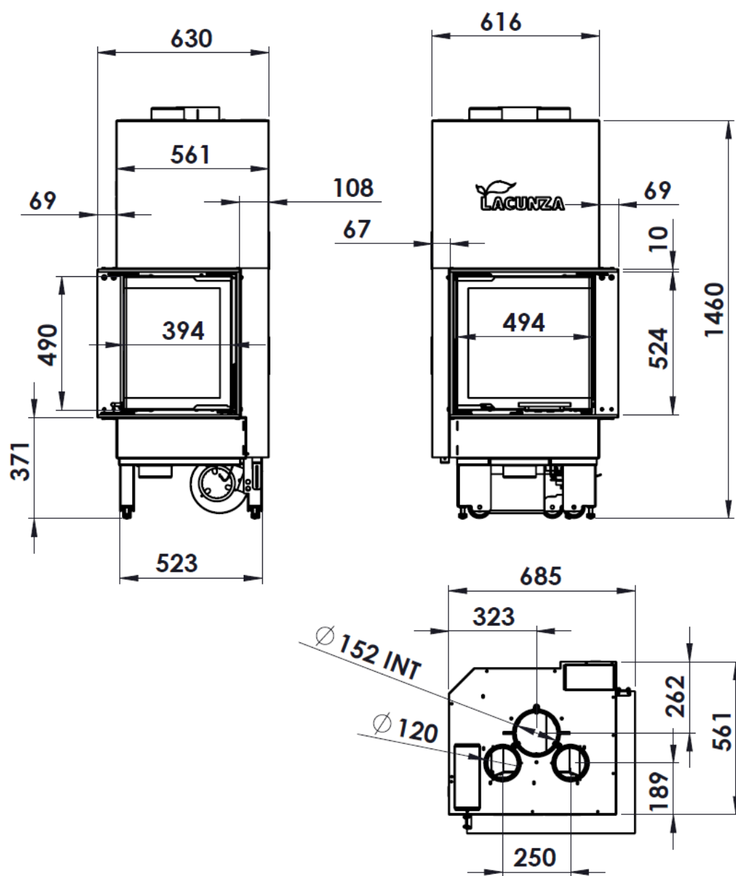
Figure n°2 - Dimensions en mm de l'appareil IZARO 60/STAR CLD
