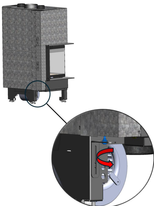
Figure n°5 - Accès pour dévisser les vis de fixation des contrepoids IZARO CLI
