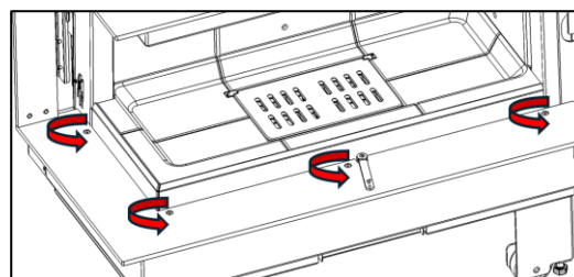
Figure n°15 - Dévissez les 8 vis qui fixent le cadre extérieur, 4 supérieurs et 4 inférieurs
