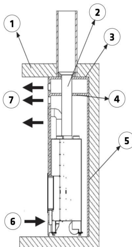
Figure n°7 - Schéma intérieur de la fermeture
