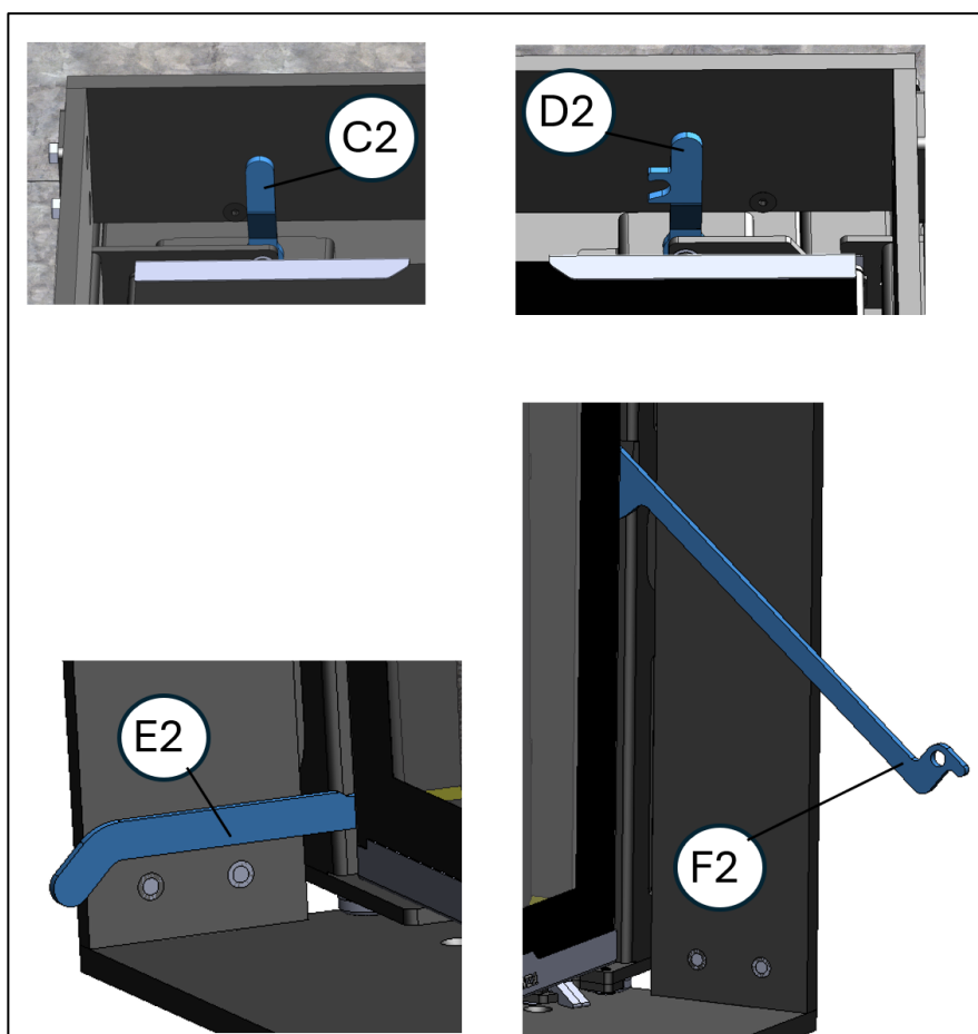
Figure n°27 - Éléments de fonctionnement de l'appareil IZARO 60 CLI
