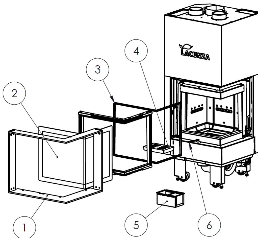
Figure n°48 - Pièces détachées Izaro 60 CLD
