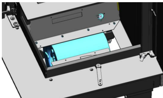
Figure n°44 - Accès à la turbine par l'intérieur de foyer
