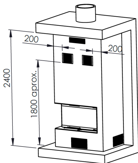
Figure n°8 - Schéma extérieur de la fermeture
