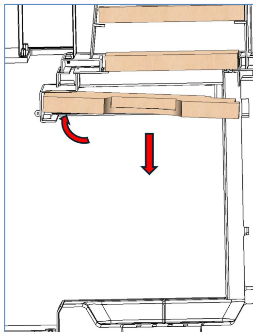
Figure n°33 - Démontage du déflecteur inférieur gauche (côté vitre latérale)
