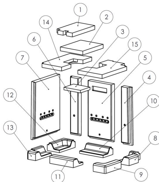
Figure n°49 - Pièces détachées foyer vermi Izaro 60 CLD
