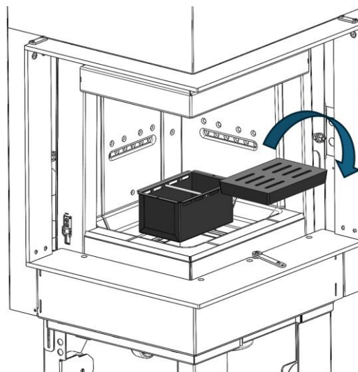
Figure n°29 - Retrait du tiroir cendrier
