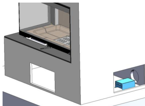
Figure n°21 - Positionnement du module de puissance devant la grille de ventilation latérale
