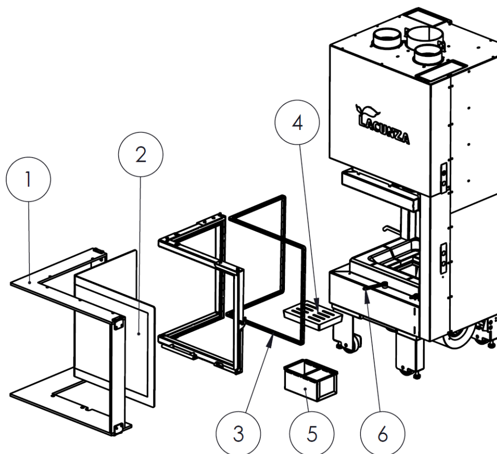
Figure n°46 - Pièces détachées Izaro 60 CLI
