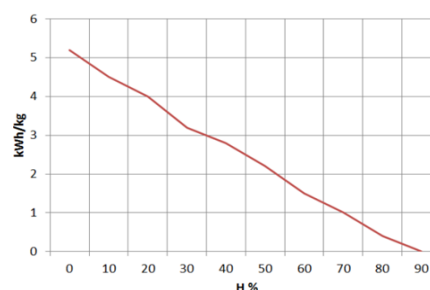
Figure n°26 - Rapport entre humidité et pouvoir calorifique du bois.
