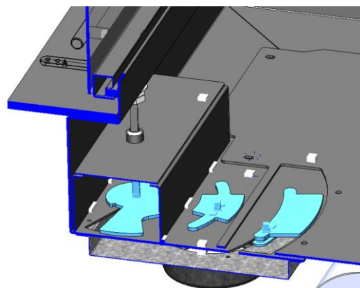
Figure n°45 - Registres amovibles
