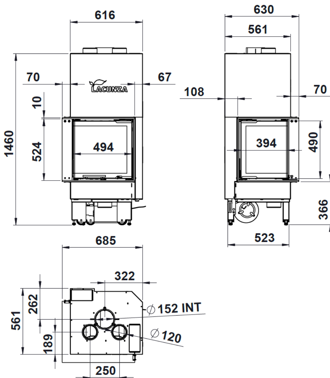
Figure n°1 - Dimensions en mm de l'appareil IZARO 60/STAR CLI
