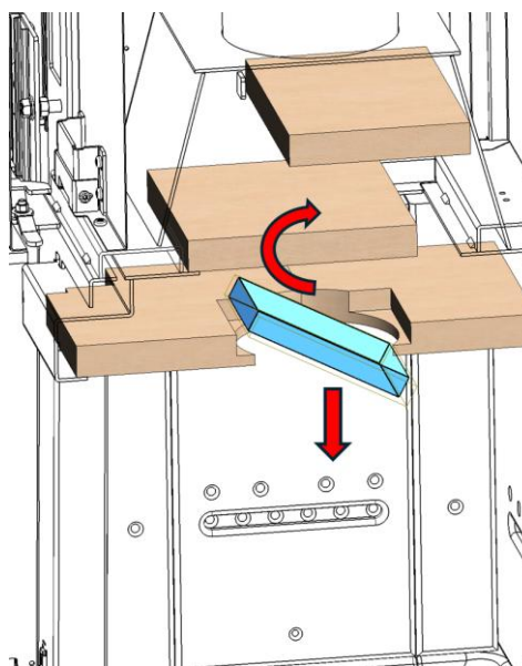
Figure n°31 - Démontage du catalyseur
