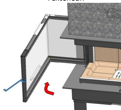
Figure n°41 - Porte ouverte horizontalement
