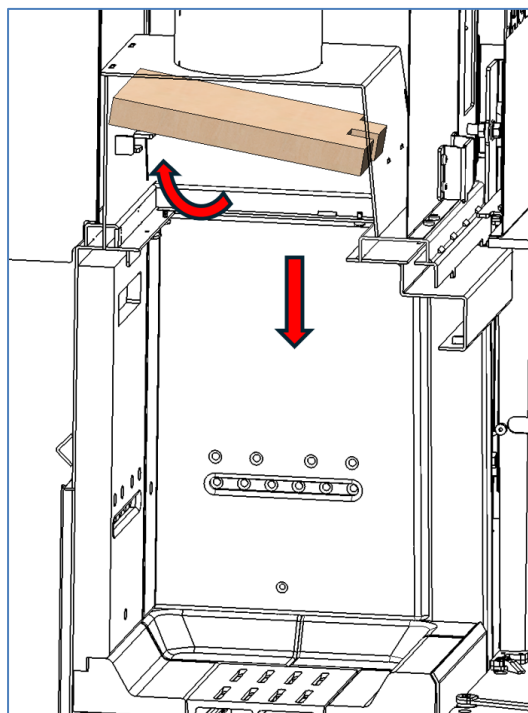
Figure n°35 - Démontage du déflecteur supérieur Izaro 60 CLI
