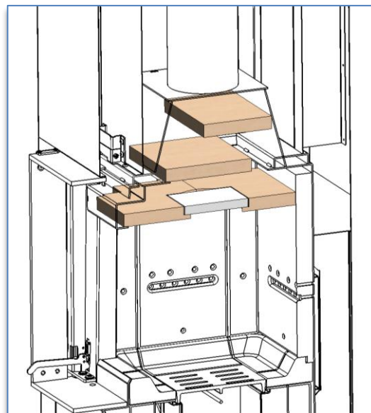
Figure n°30 - Vue de section Iزارو 60 CLI avec les déflecteurs placés
