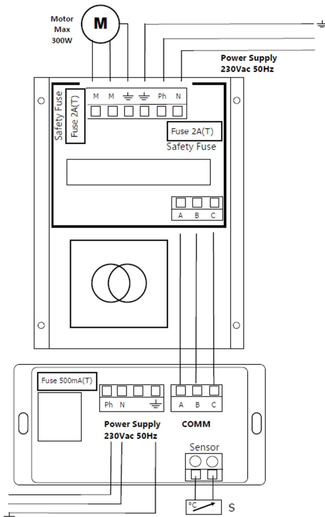
Figure n°18 - Branchements à effectuer dans le contrôleur et le module de puissance de Izaro C/V
