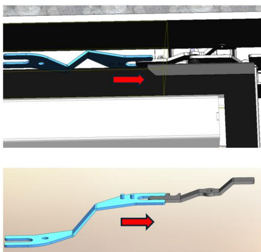
Figure n°37 - Insérer l'outil de manipulation dans le levier rotatif supérieur droit
