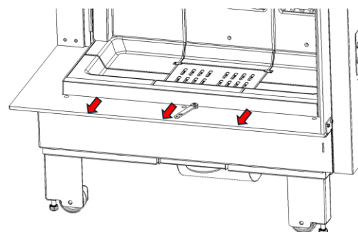
Figure n°16 - Retrait du cadre
