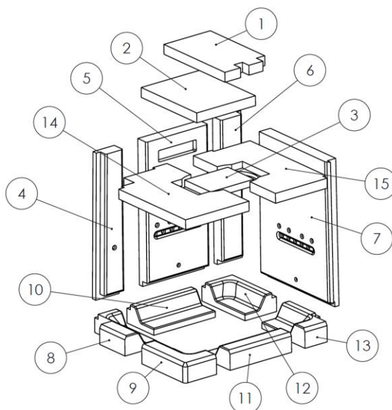
Figure n°47 - Pièces détachées foyer vermi Izaro 60 CLI
