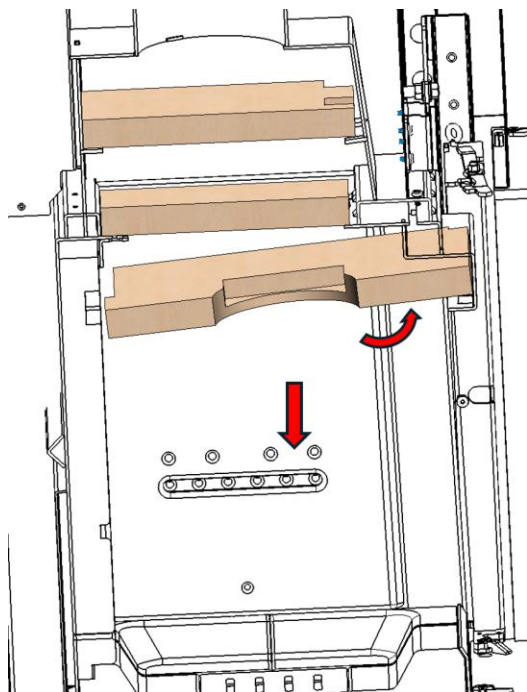
Figure n°32 - Démontage du déflecteur inférieur droit (côté opposé à la vitre latérale)
