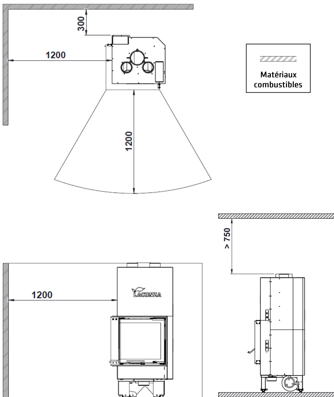
Figure n°3 - Distances de sécurité Izaro 60/STAR CLI
