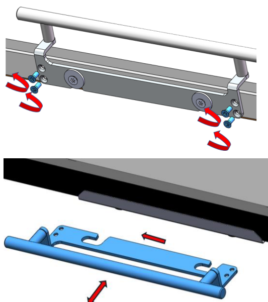
Figure n°42 - Extraction de vis et utilisation comme poignée froide
