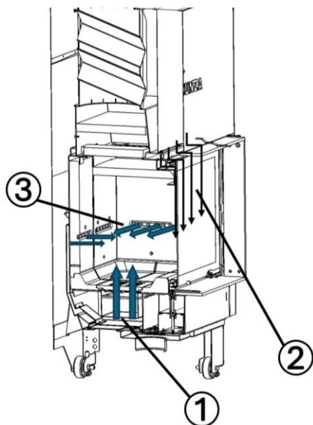
Figure n°28 - Entrées d'air de combustion
