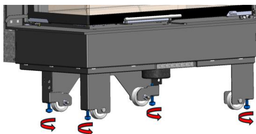
Figure n°6 - Image de 4 pieds réglables en hauteur
