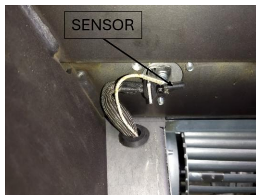
Figure n°22 - Position de la sonde de température (SENSOR) dans la sortie d'air chaud
