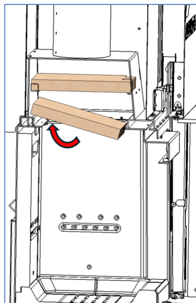
Figure n°34 - Démontage du déflecteur médium Izaro 60 CLI
