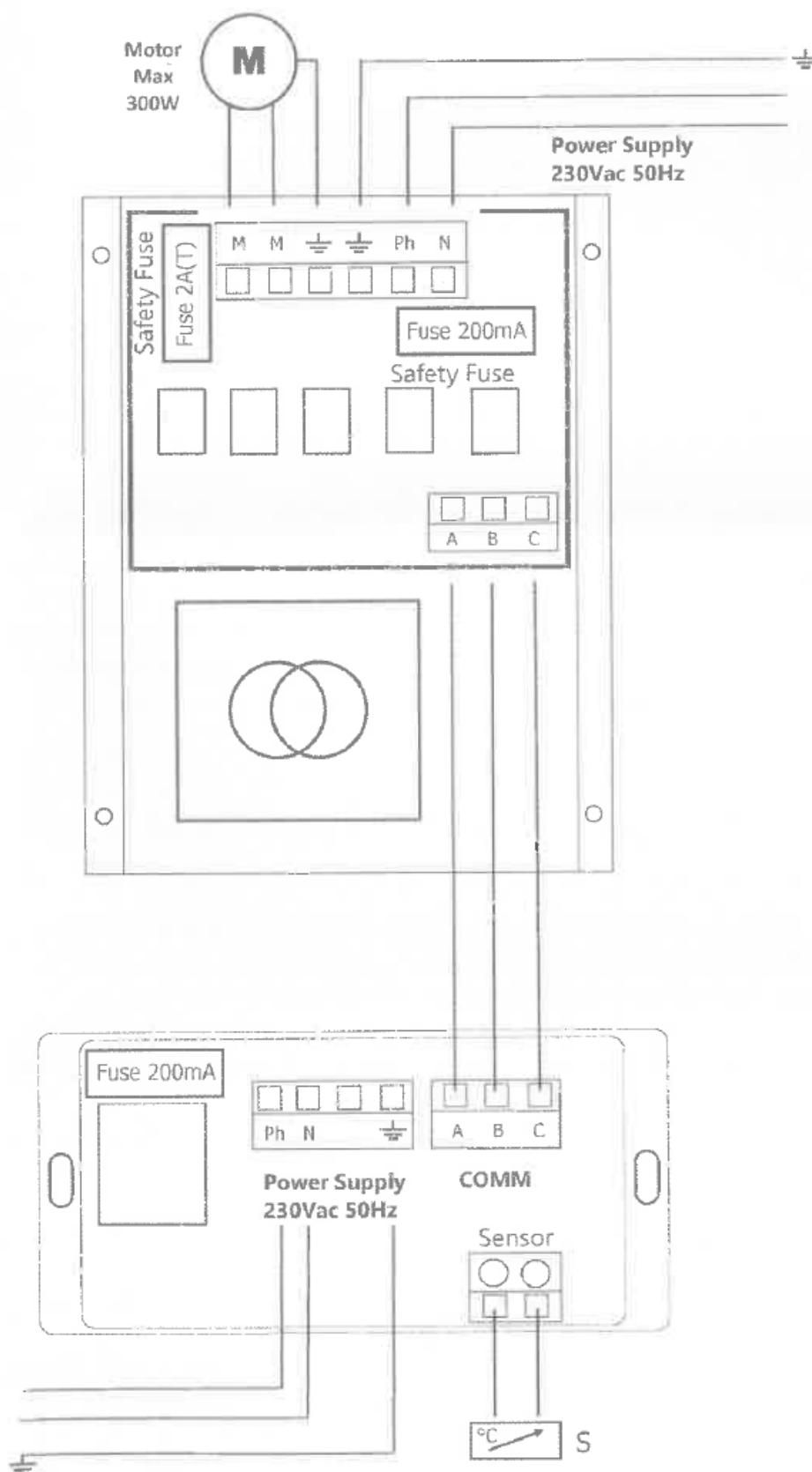
Figure n°17 - Branchements à effectuer dans le contrôleur et le module de puissance de l'Itaca eco C/V
