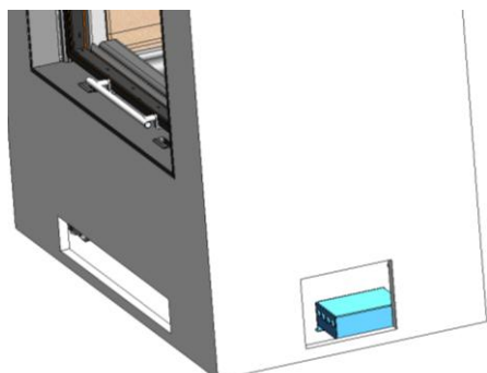
Figure n°15 - Positionnement du module de puissance devant la grille de ventilation avant
