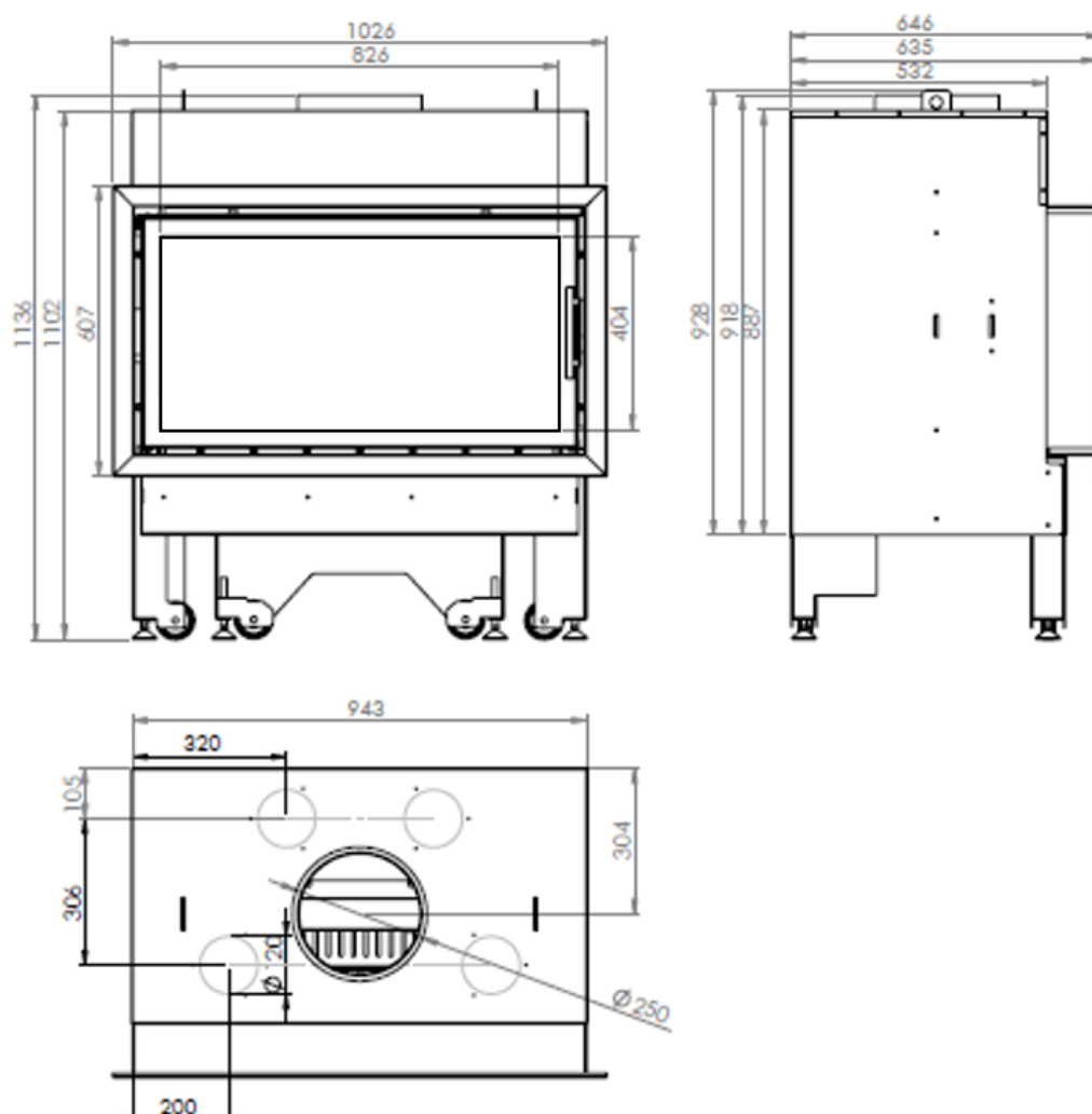
Figure n°2 - Dimensions en mm de l'appareil INCA 100
