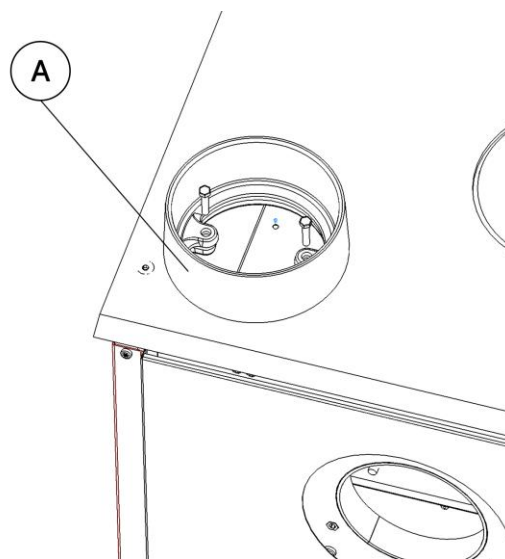
Figure n°5 - Nous plaçons la bride supérieure de sortie de fumée
