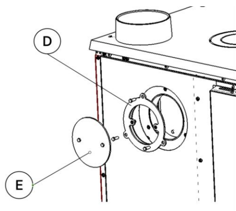
Figure n°6 - Nous plaçons l'adaptateur et le couvercle
