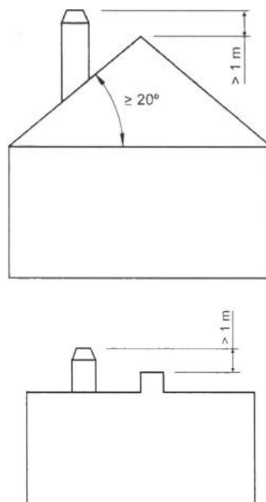
Figure n°7 - Distances depuis le haut du sommet jusqu'au faîtage du toit
