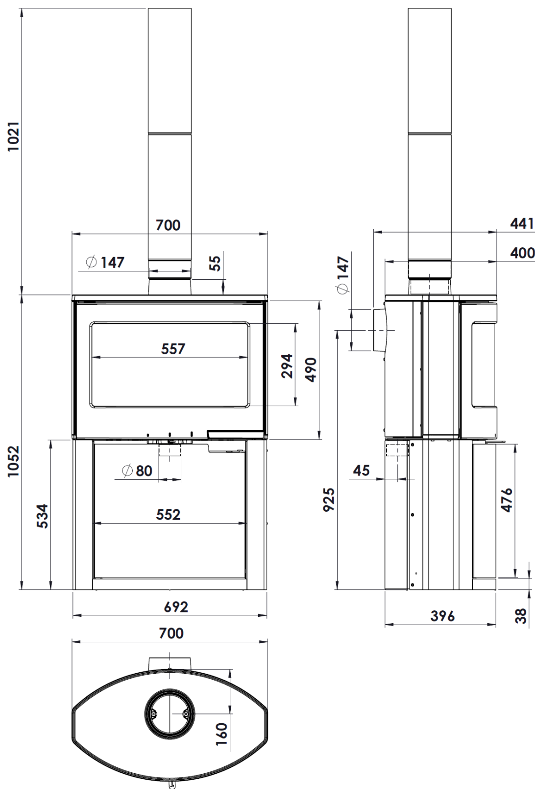
Figure n°2 - Dimensions en mm de l'appareil Bera Star
