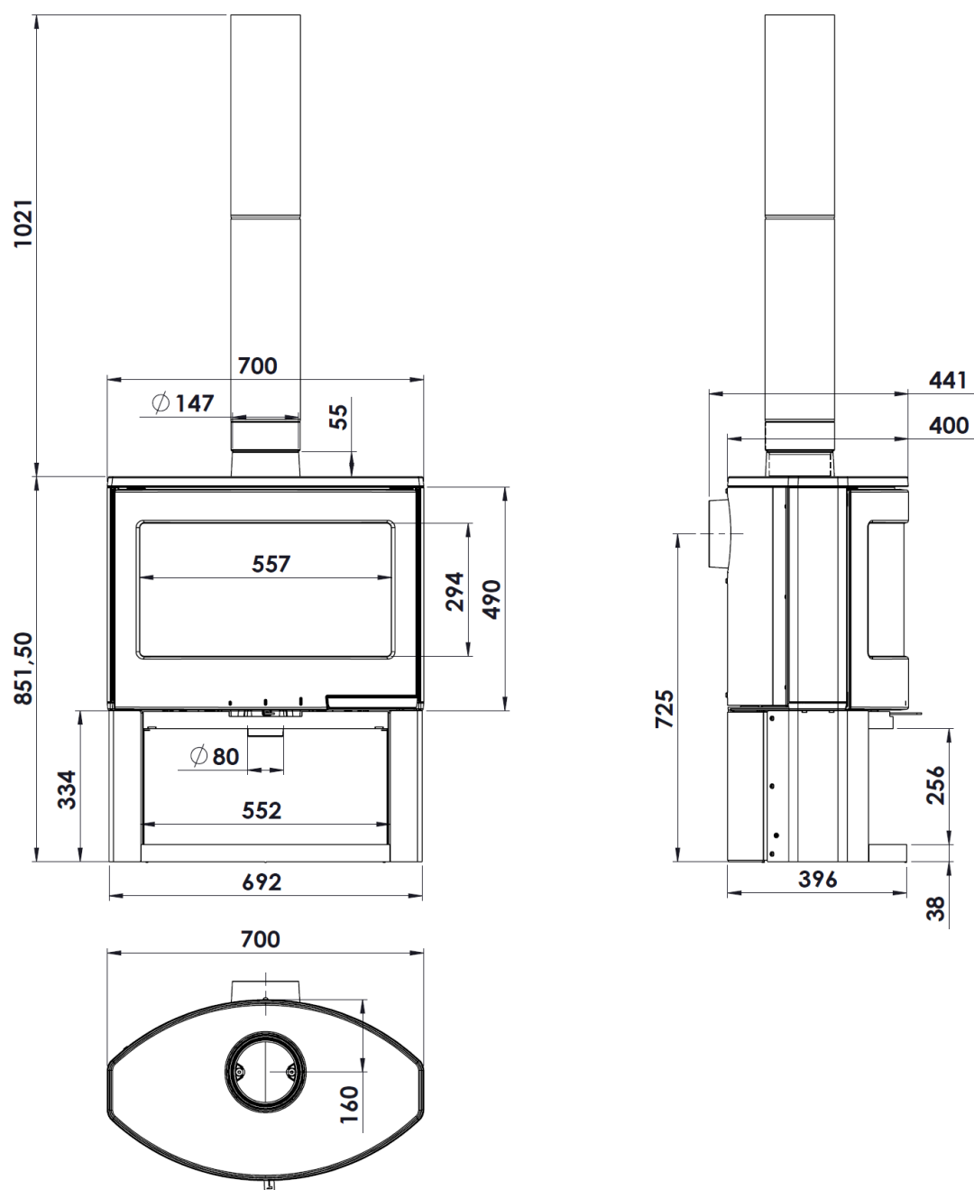
Figure n°1 - Dimensions en mm de l'appareil Dublin Star / Bristol Star
