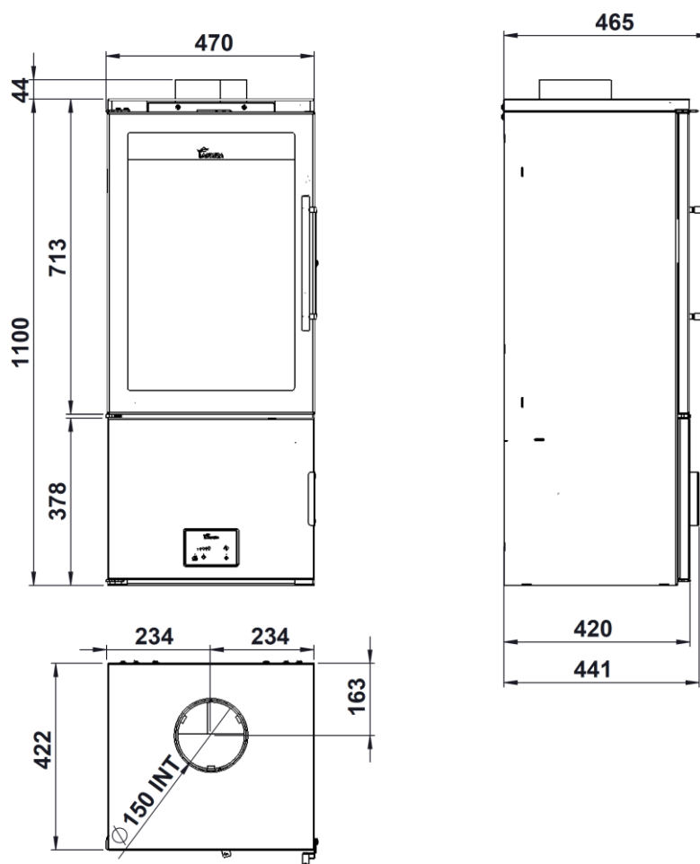
Figure n°1 - Dimensions en mm de l'appareil.
