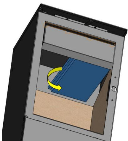
Figure n°7 - Extraction des déflecteurs en vermiculite
