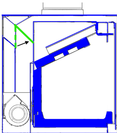
Figure n°17 - Changer la position de la tôle intérieure en la poussant vers l'intérieur.
