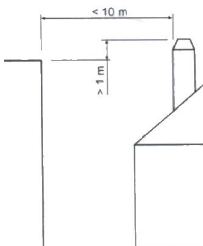
Figure n°20 - Distances entre le sommet et les objets à moins de 10m
