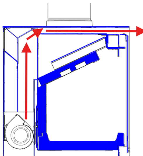
Figure n°16 - Circulation de l'air chaud sans canalisation
