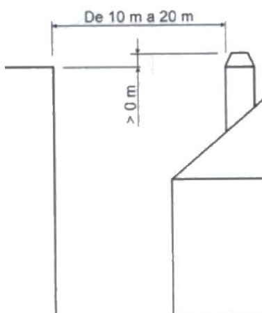
Figure n°21 - Distances entre le sommet et les objets entre 10 et 20m
