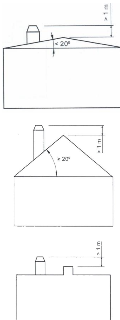
Figure n°19 - Distances depuis le haut du sommet jusqu'au faîtage du toit
