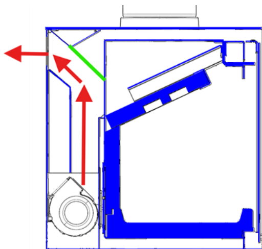
Figure n°18 - Circulation de l'air chaud avec canalisation
