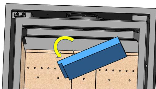
Figure n°26 - Démontage du vermiculite déflecteur plus bas
