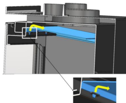
Figure n°27 - Démontage du déflecteur acier
