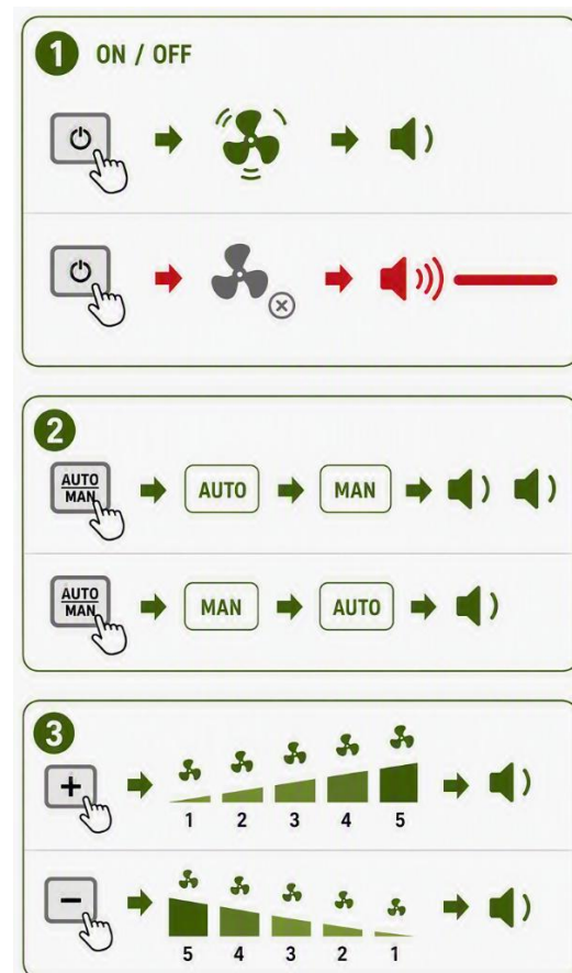
Figure n°1 - Télécommande
