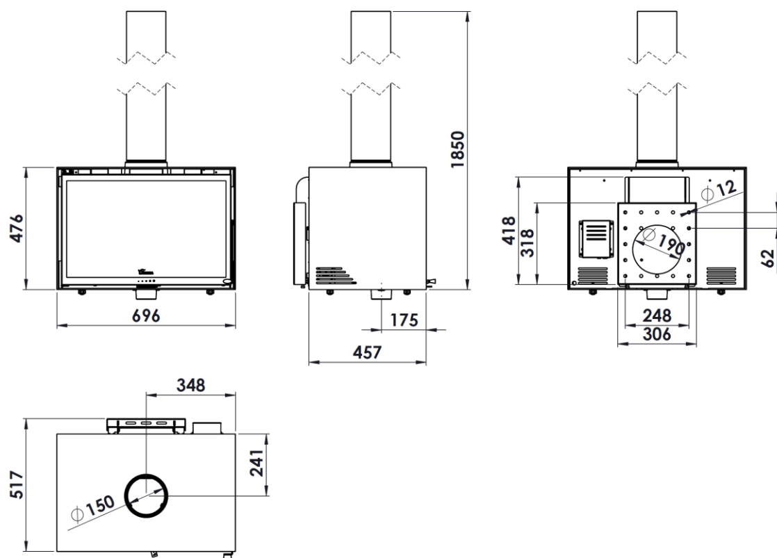
Figure n°2 - Dimensions en mm de l'appareil BAIONA 700 STAR MURAL
