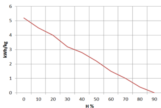
Figure n°23 - Rapport entre humidité et pouvoir calorifique du bois.
