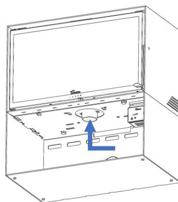
Figure n°5 - Conduction d'air pour la chambre de combustion
