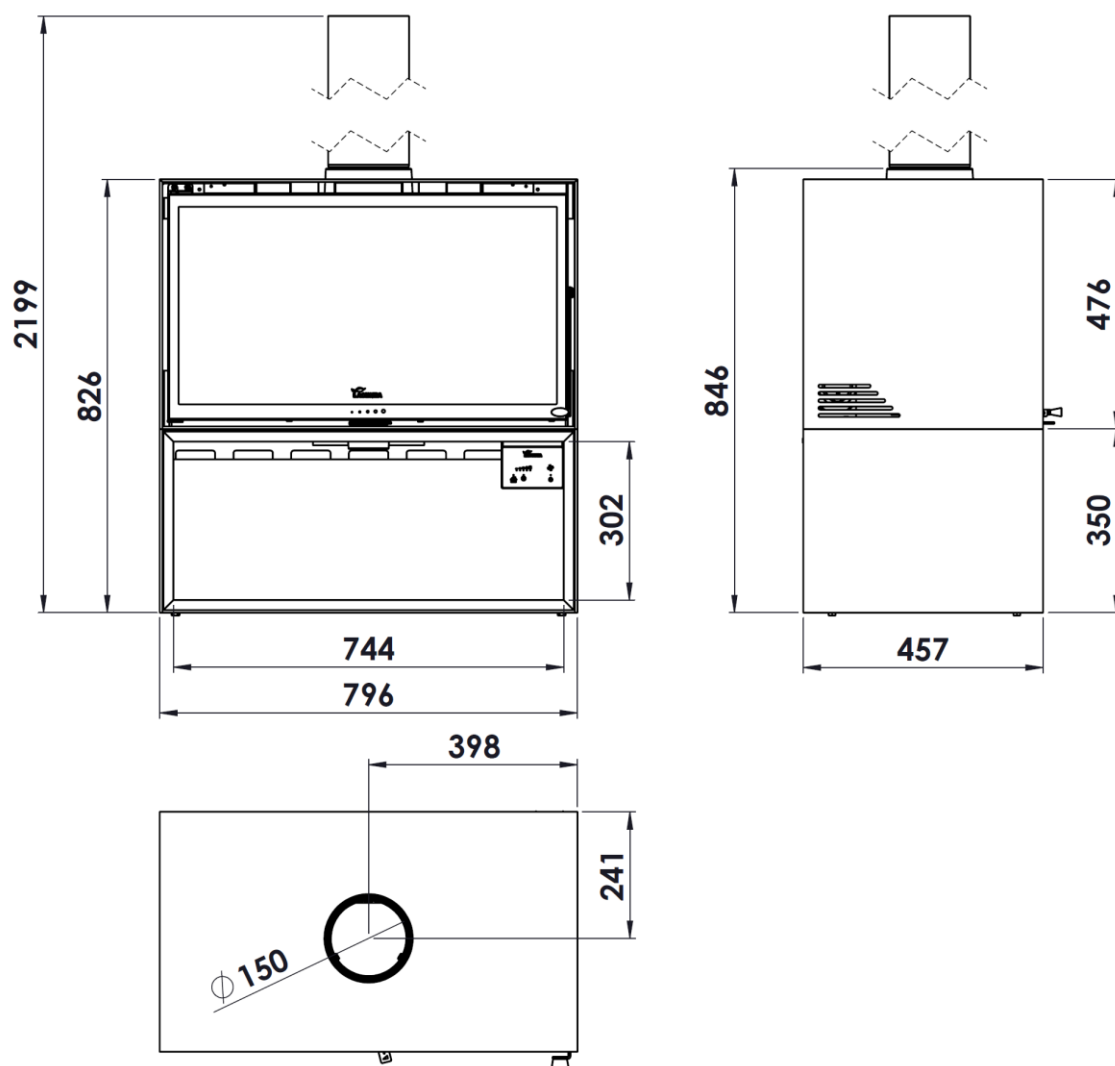
Figure n°2 - Dimensions en mm de l'appareil BAIONA 800
