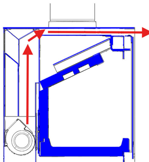
Figure n°14 - Circulation de l'air chaud sans canalisation
