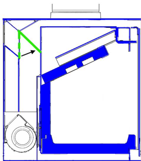
Figure n°15 - Changer la position de la tôle intérieure en la poussant vers l'intérieur.
