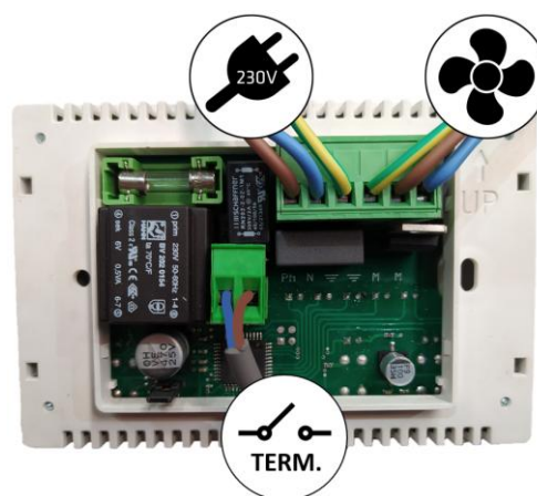
Figure n°7 - Connexions à réaliser au potentiomètre
