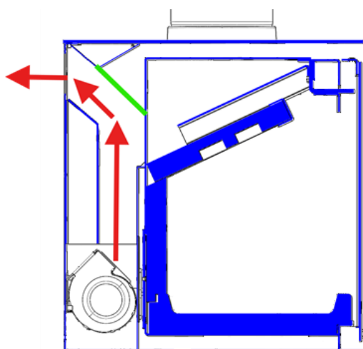
Figure n°16 - Circulation de l'air chaud avec canalisation
