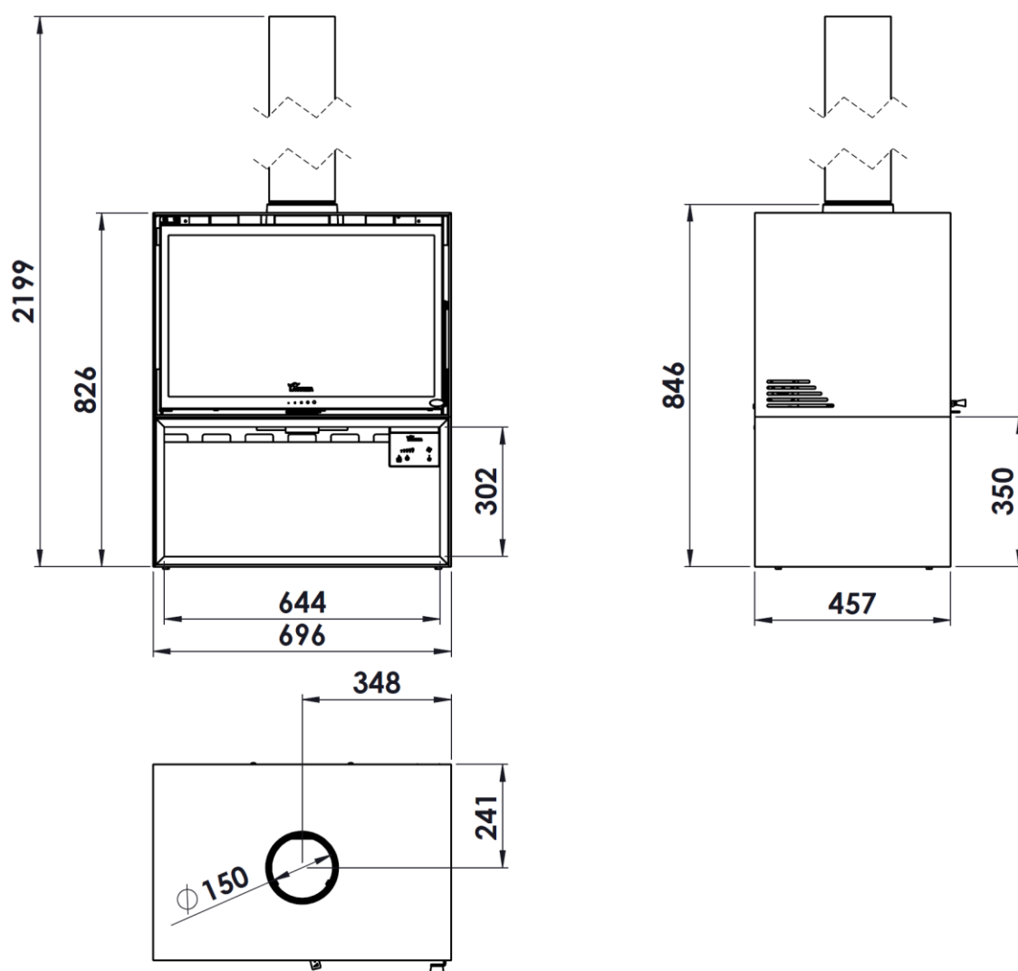
Figure n°1 - Dimensions en mm de l'appareil BAIONA 700
