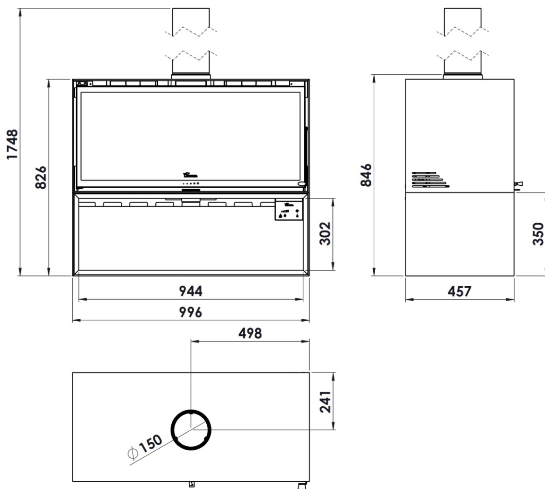
Figure n°3 - Dimensions en mm de l'appareil BAIONA 1000
