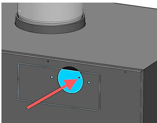
Figure n°12 - Changer la position de la tôle intérieure en la poussant vers l'intérieur.
