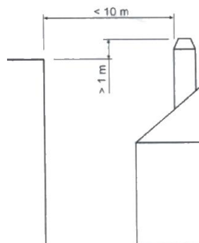
Figure n°18 - Distances entre le sommet et les objets à moins de 10m
