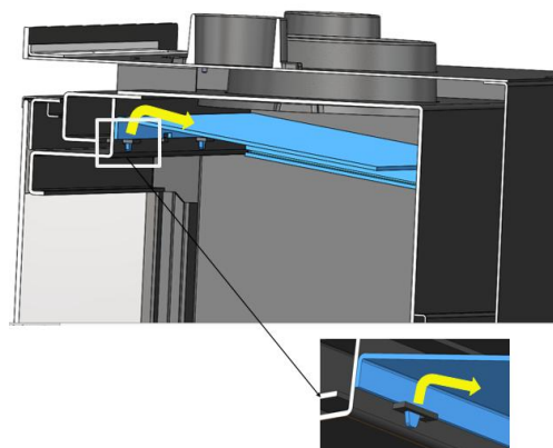
Figure n°24 - Démontage du déflecteur acier
