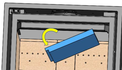
Figure n°23 - Démontage du vermiculite déflecteur plus bas
