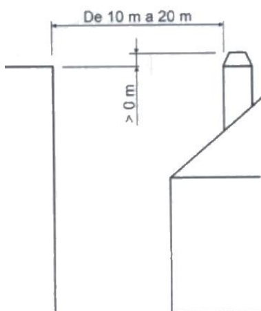
Figure n°19 - Distances entre le sommet et les objets entre 10 et 20m
