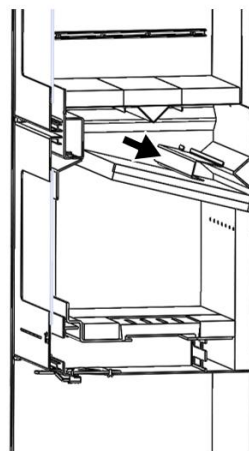
Figure n°13 - Renfort sur les déflecteurs en vermiculite
