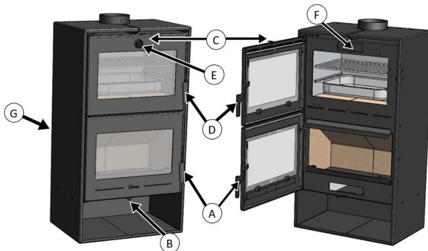
Figure n°7 - Éléments de fonctionnement de l'appareil
