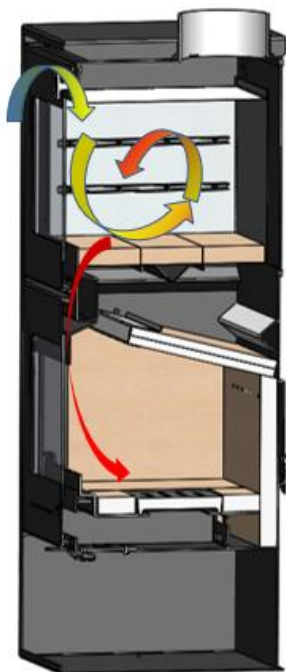
Figure n°8 - Système d'extraction de buée
