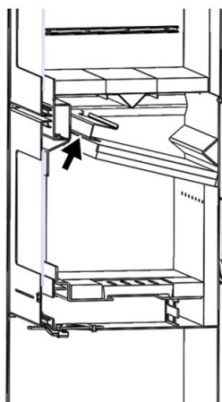
Figure n°12 - Rotation du renfort en acier inoxydable
