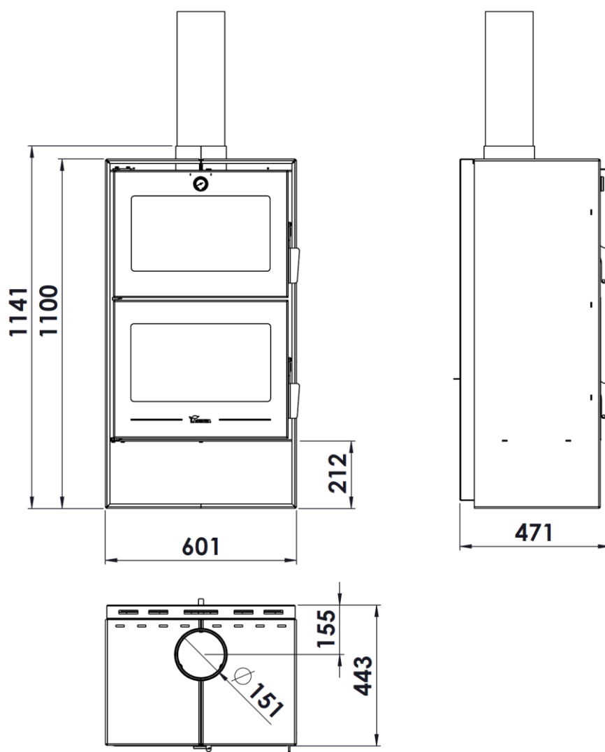
Figure n°1 - Dimensions en mm de l'appareil ALTEA
