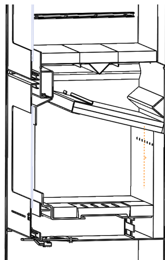
Figure n°17 - Renfort d'acier inoxydable sur la position ouverte
