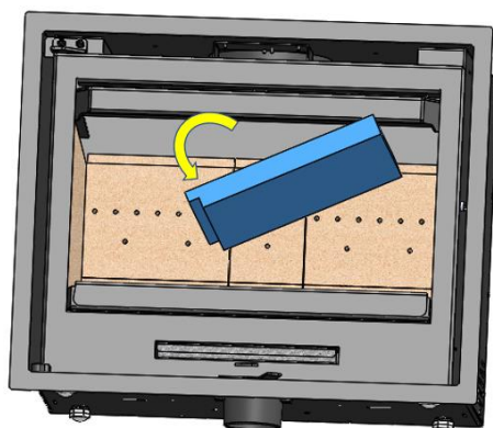
Figure n°8 - Démontage du vermiculite déflecteur plus bas
