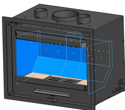
Figure n°8 - Démontage du vermiculite déflecteur plus bas
