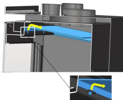
Figure n°9 - Démontage du déflecteur acier
