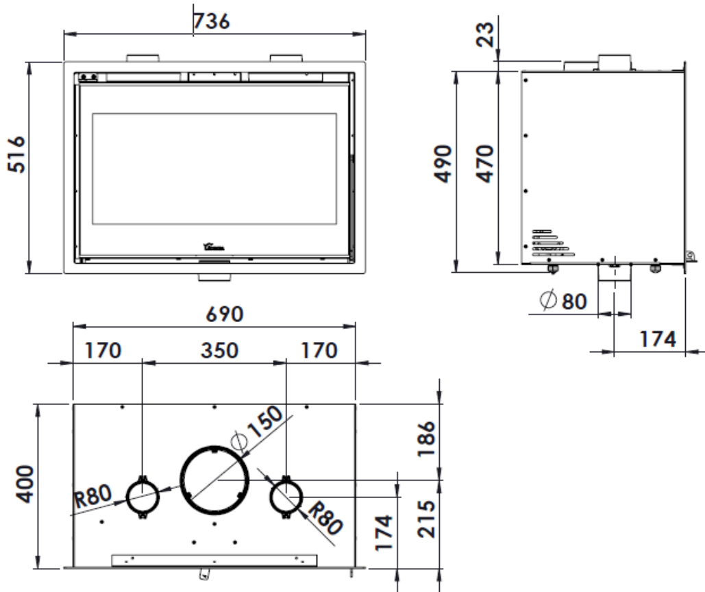
Figure n°3 - Dimensions en mm de l'appareil ADOUR 700
