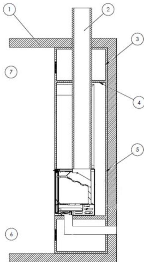
Figure n°6 - Schéma intérieur de la fermeture
