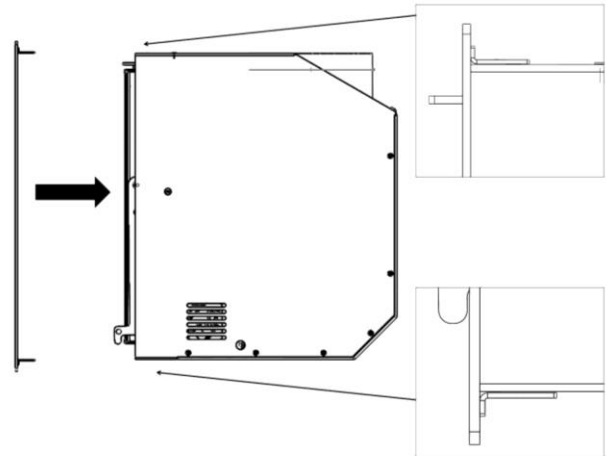
Figure n°14 - Passez l'encadrement par l'intérieur
