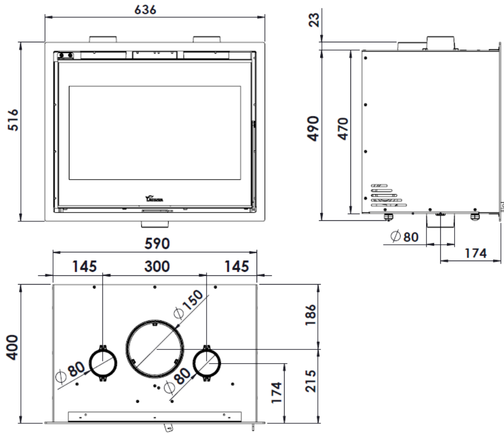
Figure n°2 - Dimensions en mm de l'appareil ADOUR 600
