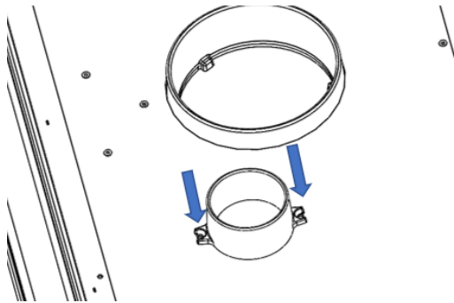
Figure n°12 - Vissez la tuyère sur la partie arrière
