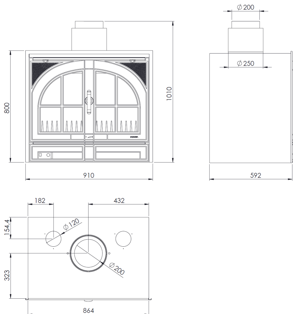
Figure n°2 - Dimensions en mm de l'appareil Abodi
