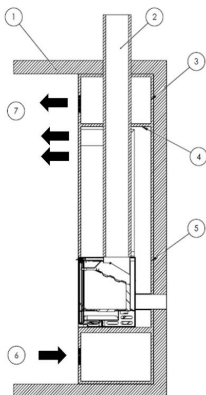
Figure n°4 - Schéma intérieur de la fermeture
