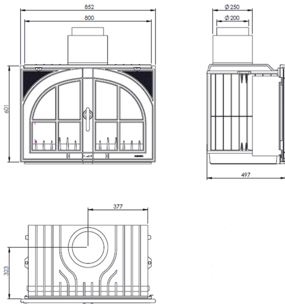
Figure n°1 - Dimensions en mm de l'appareil Sara
