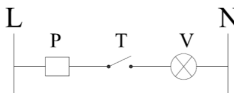
Figure n°13 - Schéma électrique
