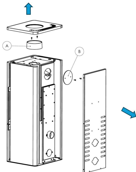
Figura n°5 - Intercambia i componenti (A) e (B) per l'uscita fumi posteriore
