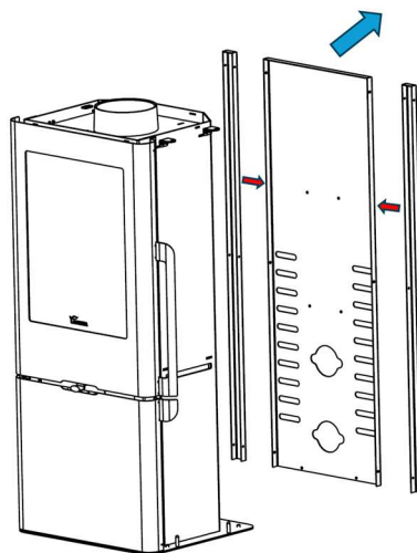
Figura n°25 - Paso 3. Smontare il doppio pannello posteriore e montare i pezzi di riempimento
