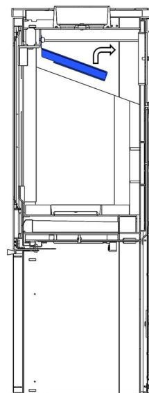
Figura n°17 - Smontaggio del deflettore in acciaio
