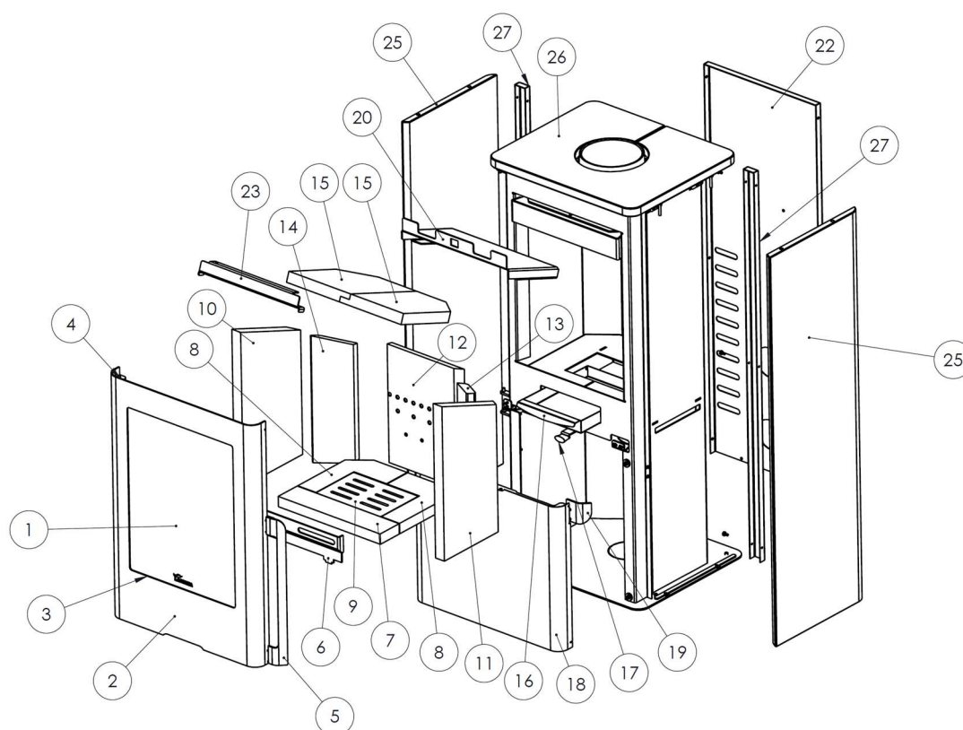
Figura n°2 - Pezzi MAYA Vision
