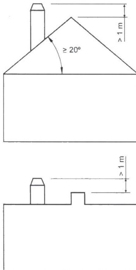
Figura n°9 - Distanza tra la finitura e il colmo del tetto
