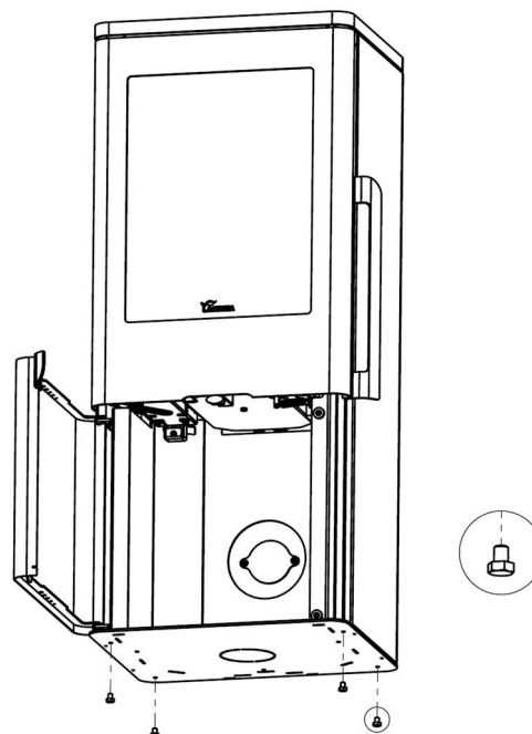
Figura n°18 - Installazione dei piedini di livellamento
