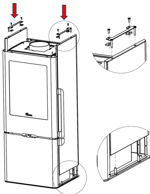
Figura n°31 - Paso 9. Posizionare i fianchi in pietra serpentino e fissarli con i supporti
