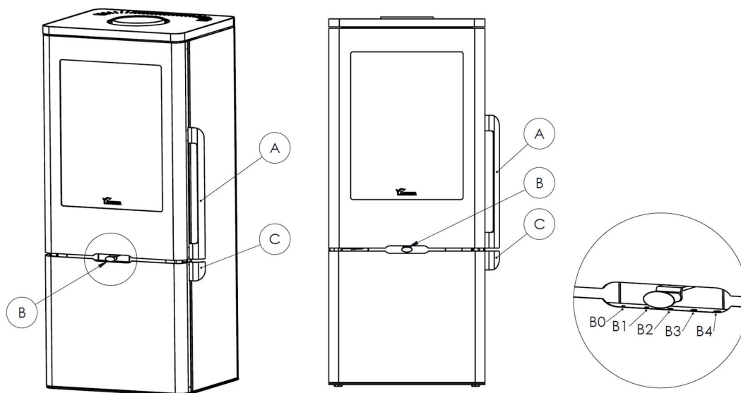
Figura n°13 - Elementi di funzionamento dell'apparecchio
