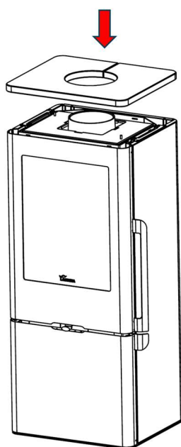
Figura n°32 - Paso 10. Posizionare il piano in pietra serpentino
