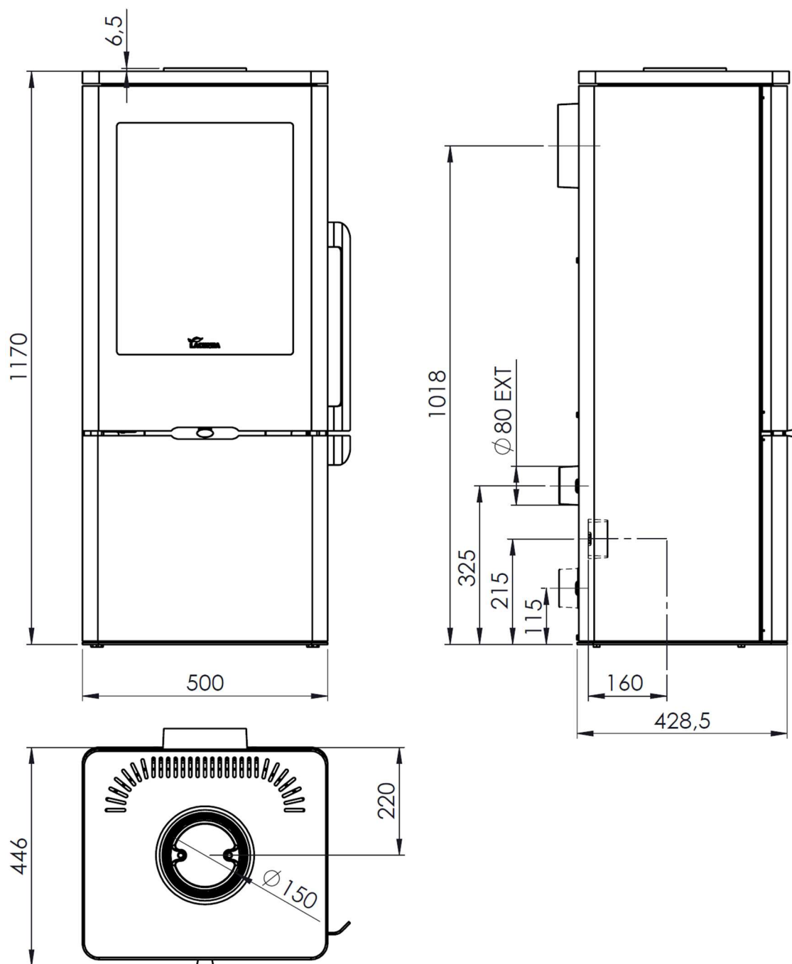
Figura n°1 - Dimensioni in mm dell'apparecchio VELA
