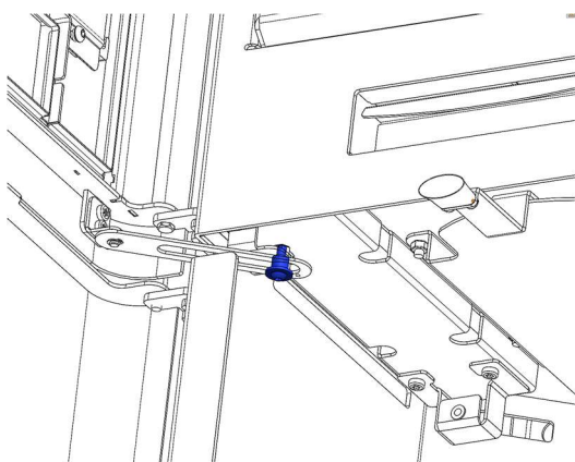
Figura n°20 - Passo 2. Smontare l'asse
