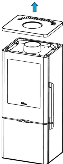
Figura n°23 - Paso 1. Smontare il piano superiore
