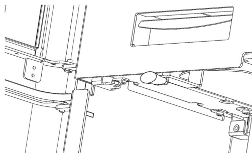
Figura n°22 - Passo 4. Rimuovere il meccanismo
