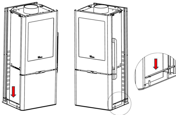
Figura n°29 - Paso 7. Montare gli spessori laterali in pietra serpentino
