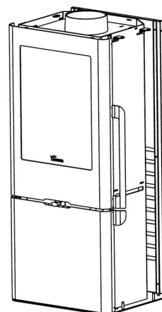
Figura n°26 - Paso 4. Montare il doppio pannello posteriore
