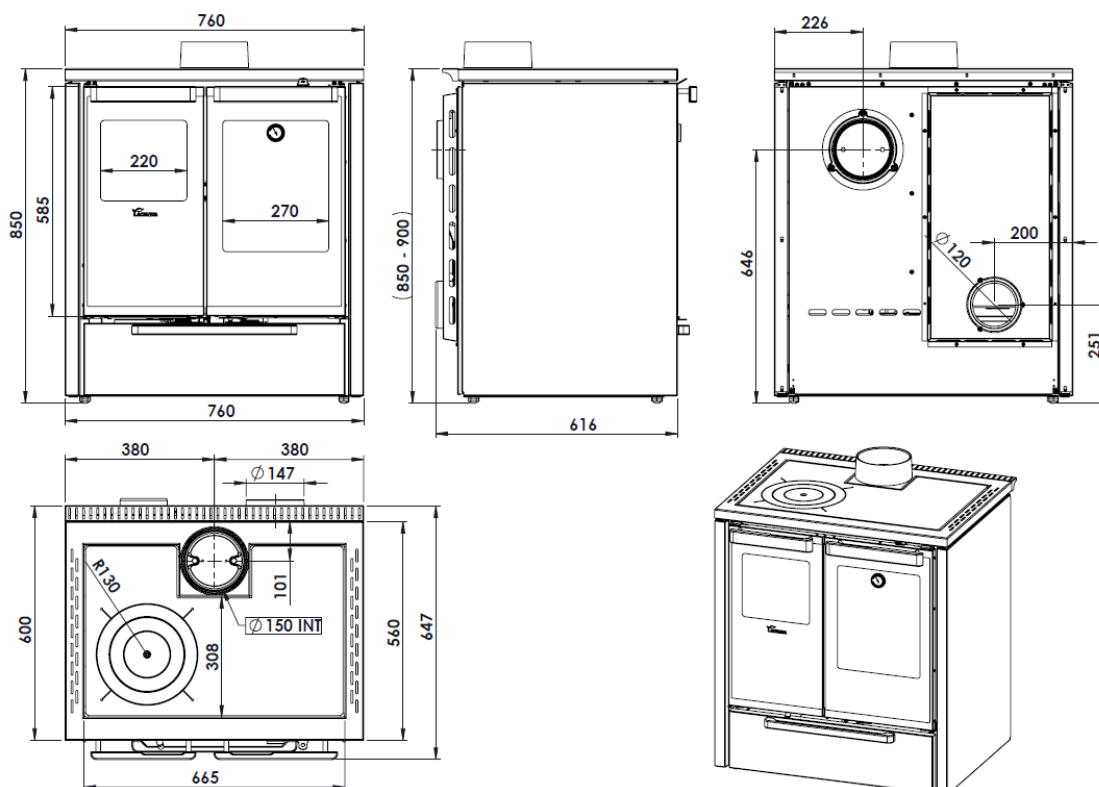
Figura n°1 - Dimensioni in mm dell'apparecchio TERRA 5T, S-SUP CEN Inox
