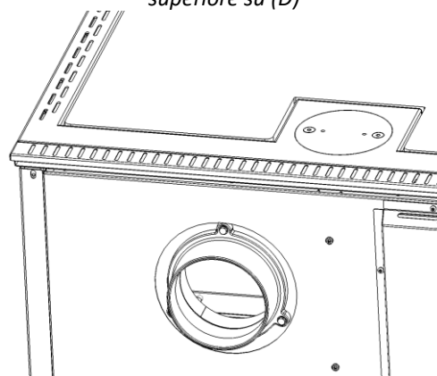
Figura n°9 - Posizioniamo la copertura superiore su (D)
