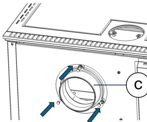
Figura n°8 - Posizioniamo la l'uscita fumo posteriore (C).
