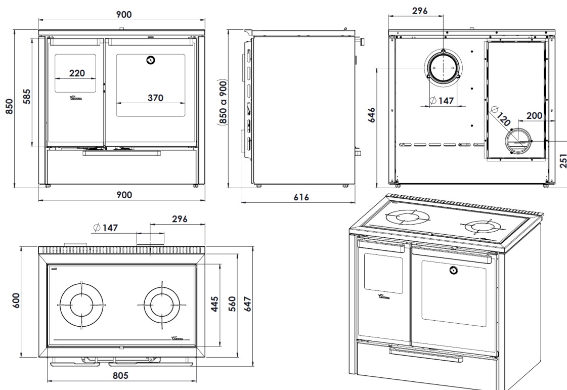
Figura n°4 - Dimensioni in mm dell'apparecchio TERRA 7T Super V
