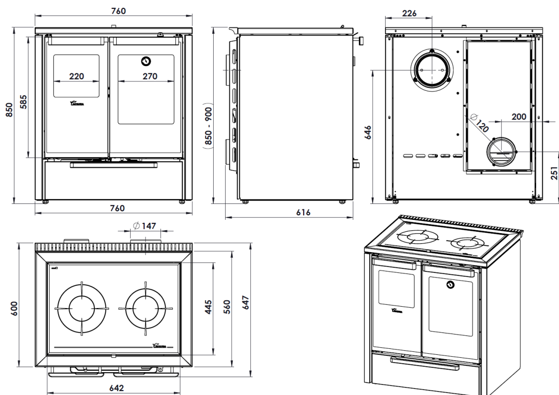
Figura n°2 - Dimensioni in mm dell'apparecchio TERRA 5T Super V
