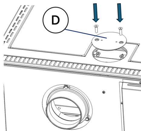
Figura n°9 - Posizioniamo la copertura superiore su (D)
