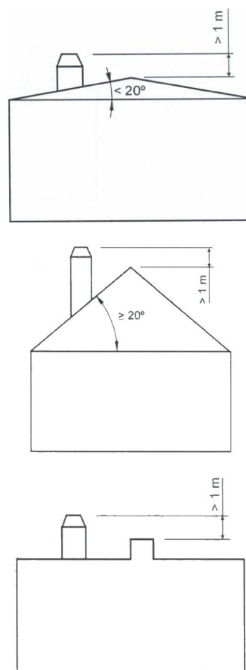
Figura n°12 - Distanza tra la finitura e il colmo del tetto
