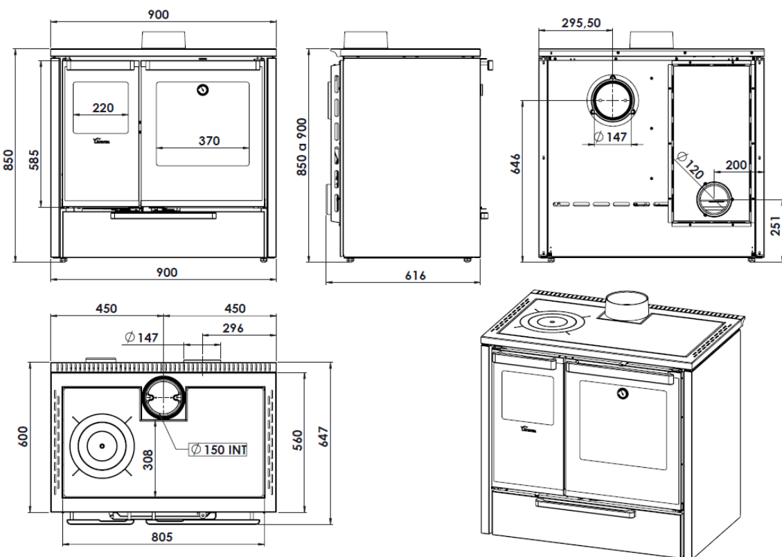
Figura n°3 - Dimensioni in mm dell'apparecchio TERRA 7T S-SUP CEN Inox
