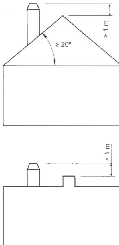
Figura n°11 - Distanza tra la finitura e il colmo del tetto
