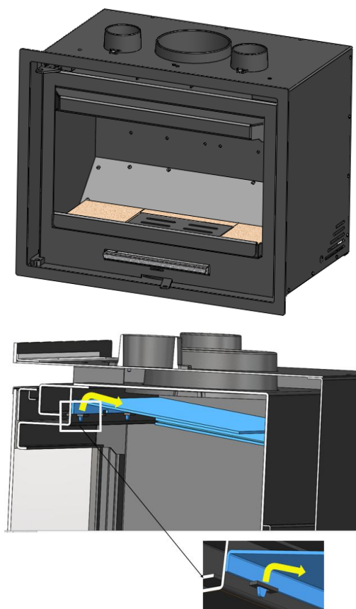
Figura n°11 - Smontaggio del deflettore superiore in acciaio
