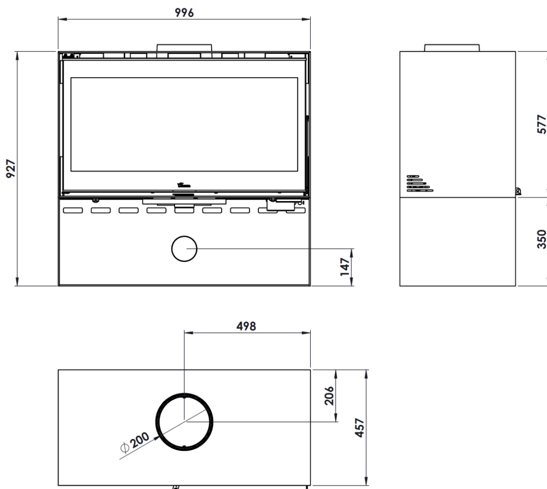
Figura n°3 - Dimensioni in mm dell'apparecchio ROMA 1000
