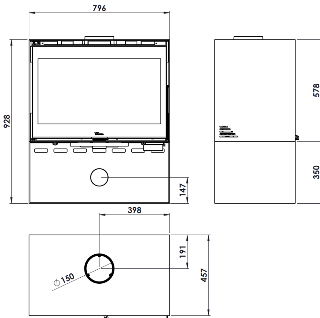
Figura n°2 - Dimensioni in mm dell'apparecchio ROMA 800
