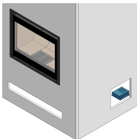
Figura n°2 - Posizionare la custodia del regolatore davanti alla bocchetta laterale
