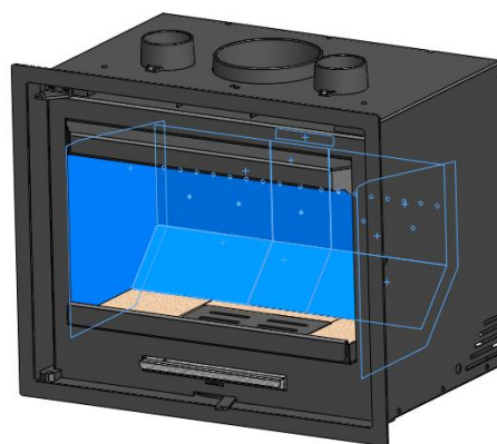
Figura n°10 - Smontaggio di deflettori inferiori
