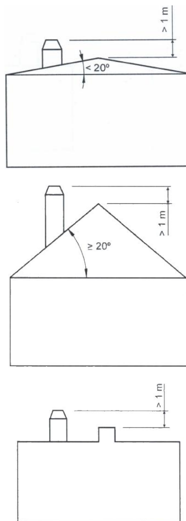
Figura n°3 - Distanza tra la finitura e il colmo del tetto
