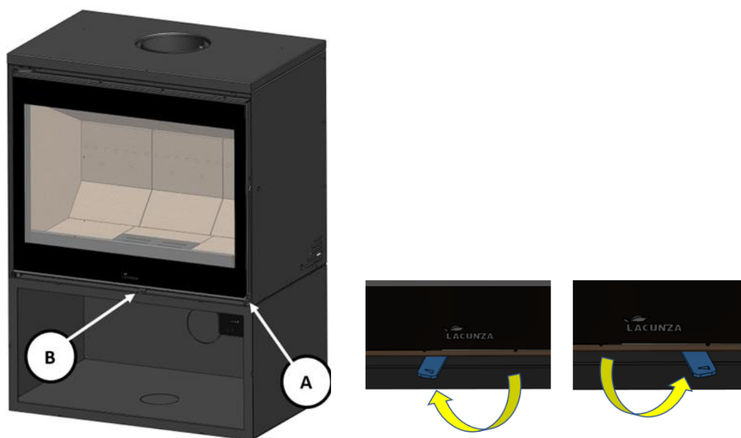
Figura n°7 - Elementi di funzionamento dell'apparecchio
