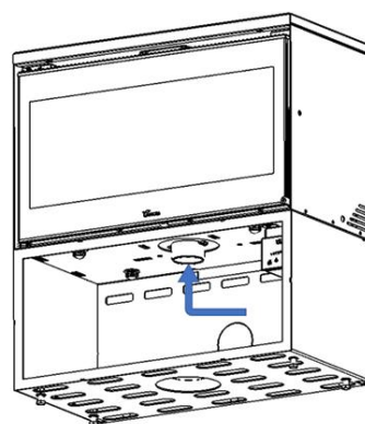
Figura n°5 - l'aria per la combustione direttamente dall'esterno
