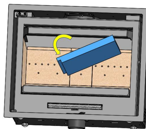
Figura n°10 - Smontaggio di deflettori inferiori
