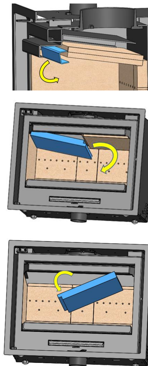
Figura n°12 - Smontaggio di deflettori inferiori
