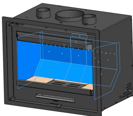
Figura n°12 - Smontaggio di deflettori inferiori
