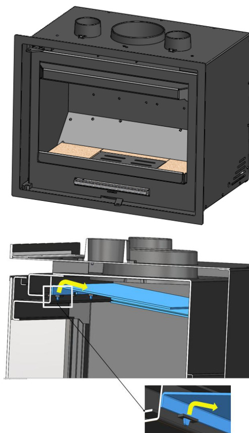
Figura n°13 - Smontaggio del deflettore superiore in acciaio
