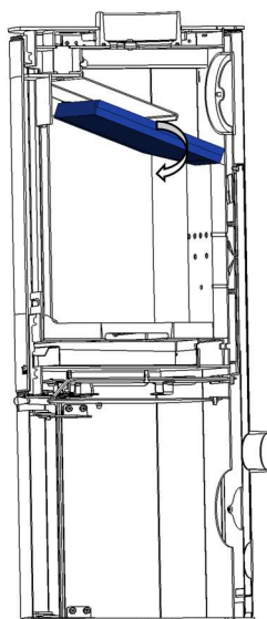
Figura n°17 - Estrazione della vermiculite
