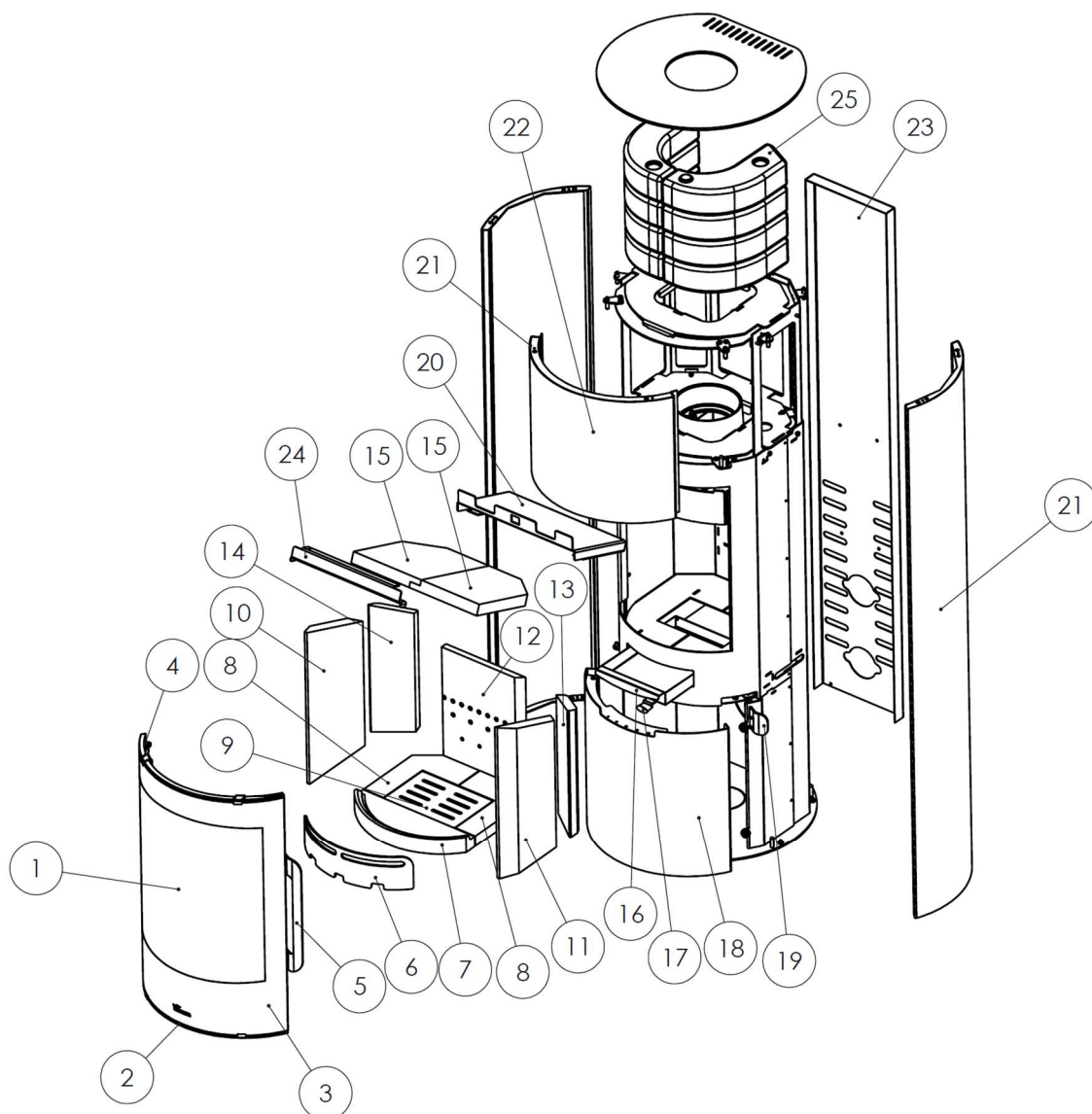
Figura nº4 - Pezzi MAYA ACU Vision
