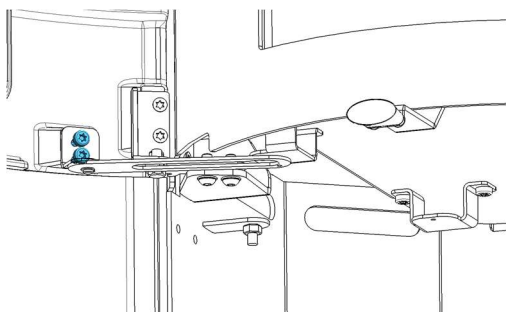
Figura n°22 - Passo 3. Rimuovere le viti di supporto della porta
