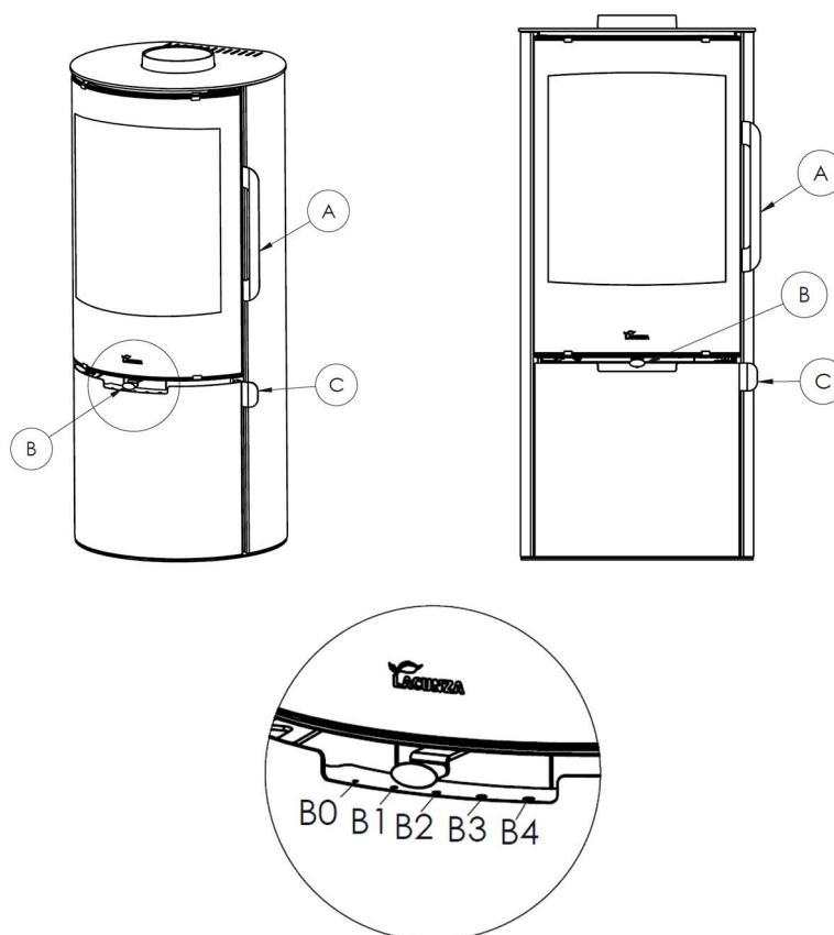
Figura n°14 - Elementi di funzionamento dell'apparecchio
