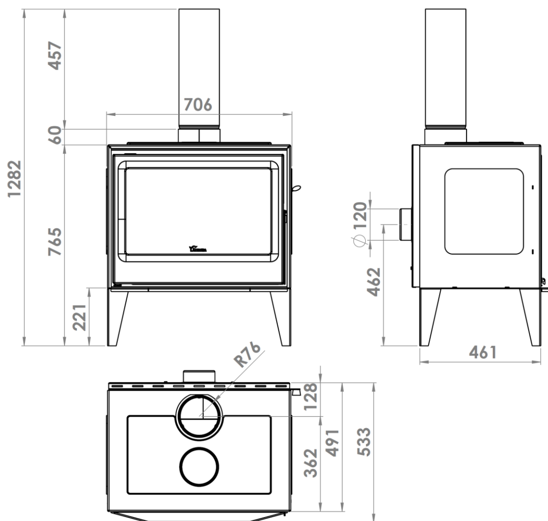
Figura n°1 - Dimensioni in mm dell'apparecchio MARTINA STAR
