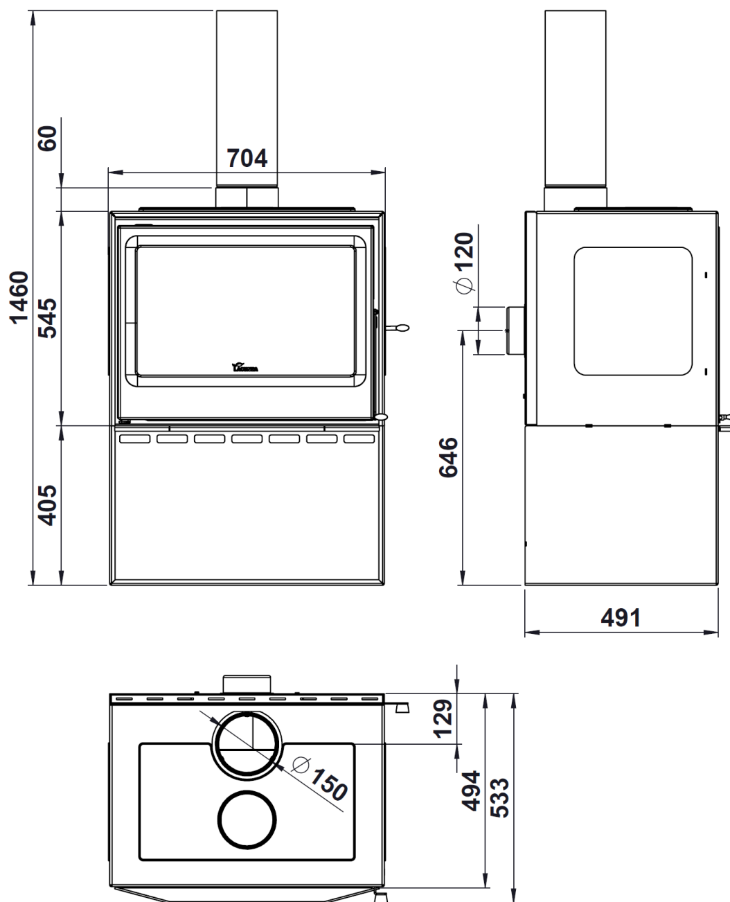
Figura n°2 - Dimensioni in mm dell'apparecchio MARTINA L STAR
