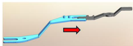
Figura n°39 - Inserire l'utensile per i perni apertura pulizia vetro porta
