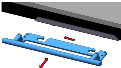
Figura n°44 - Estrazione delle viti e utilizzo come "maniglia fredda" per la maniglia
