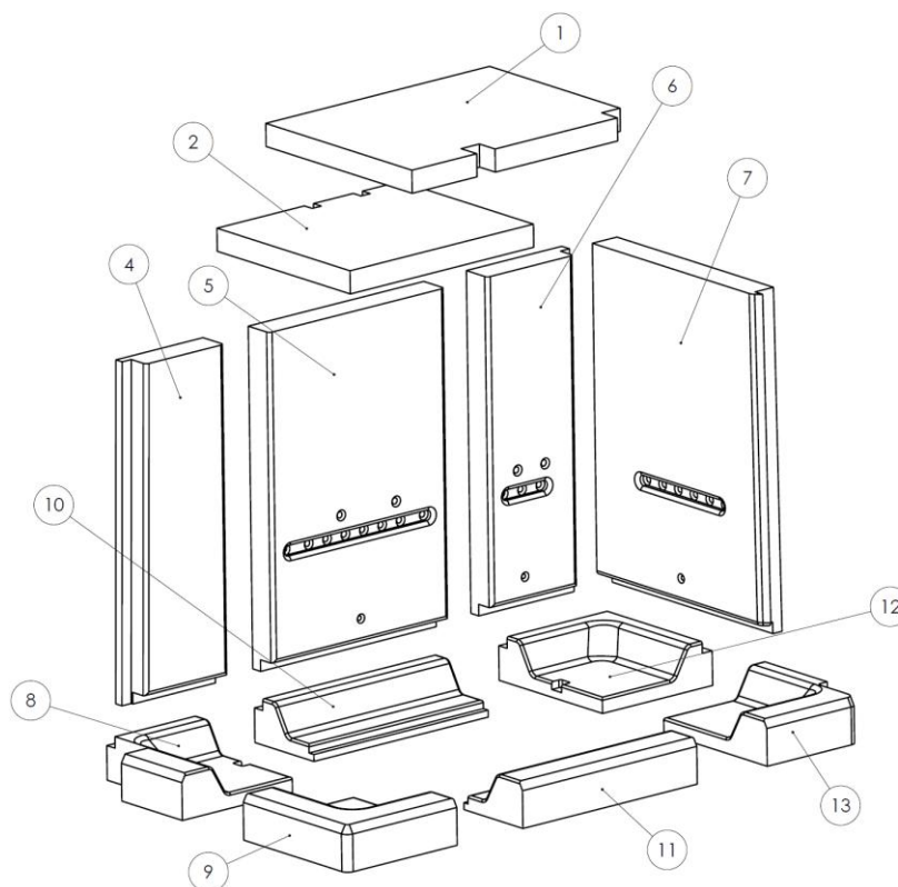
Figura n°49 - Vista esplosa vermiculite IZARO 80 CLI
