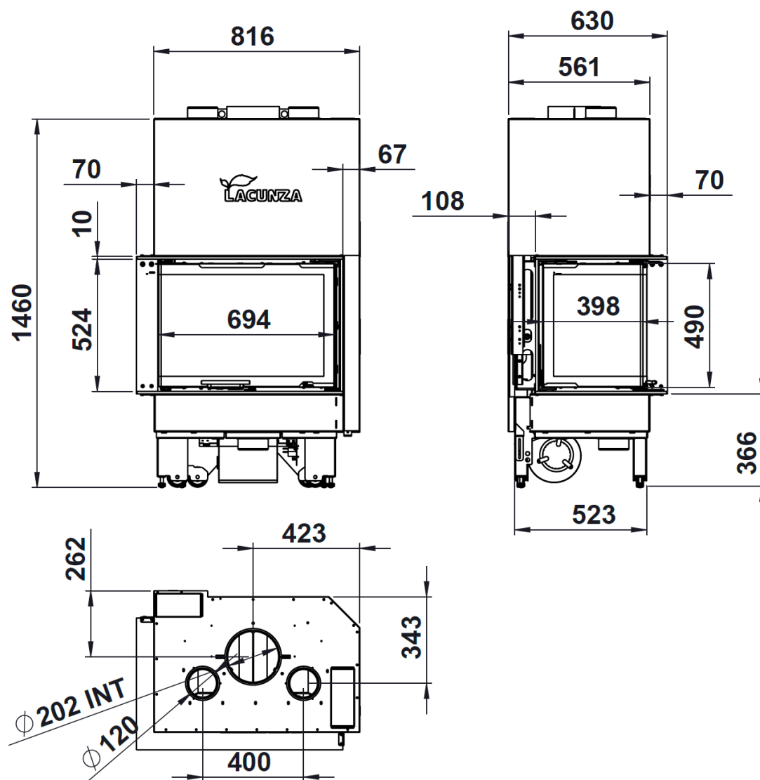
Figura n°1 - Dimensioni in mm dell'apparecchio IZARO 80 CLI
