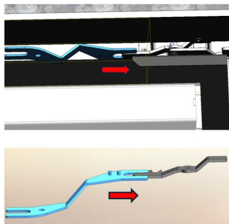
Figura n°39 - Inserirlo l'utensile per i perni apertura pulizia vetro porta
