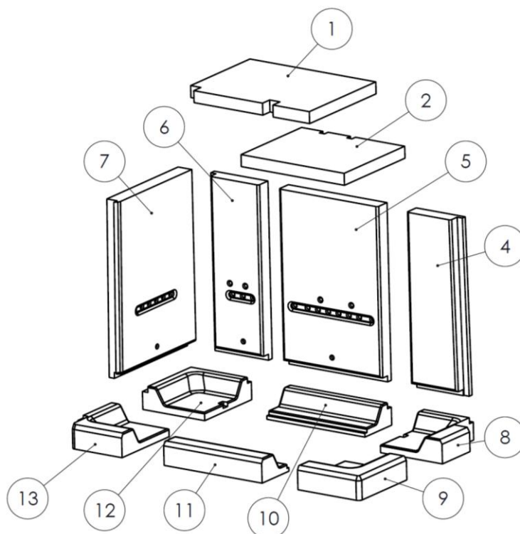
Figura n°52 - Pezzi principali vermi IZARO 80 CLD
