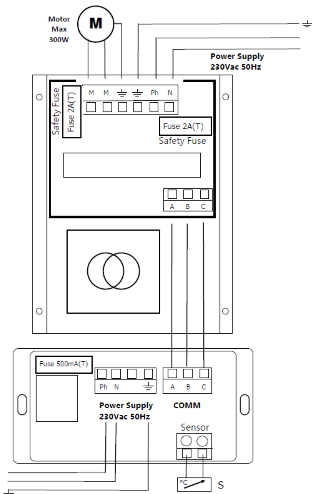
Figura n°20 - Collegamenti da effettuare nel controllore e nel modulo di potenza dell'izaro C/V
