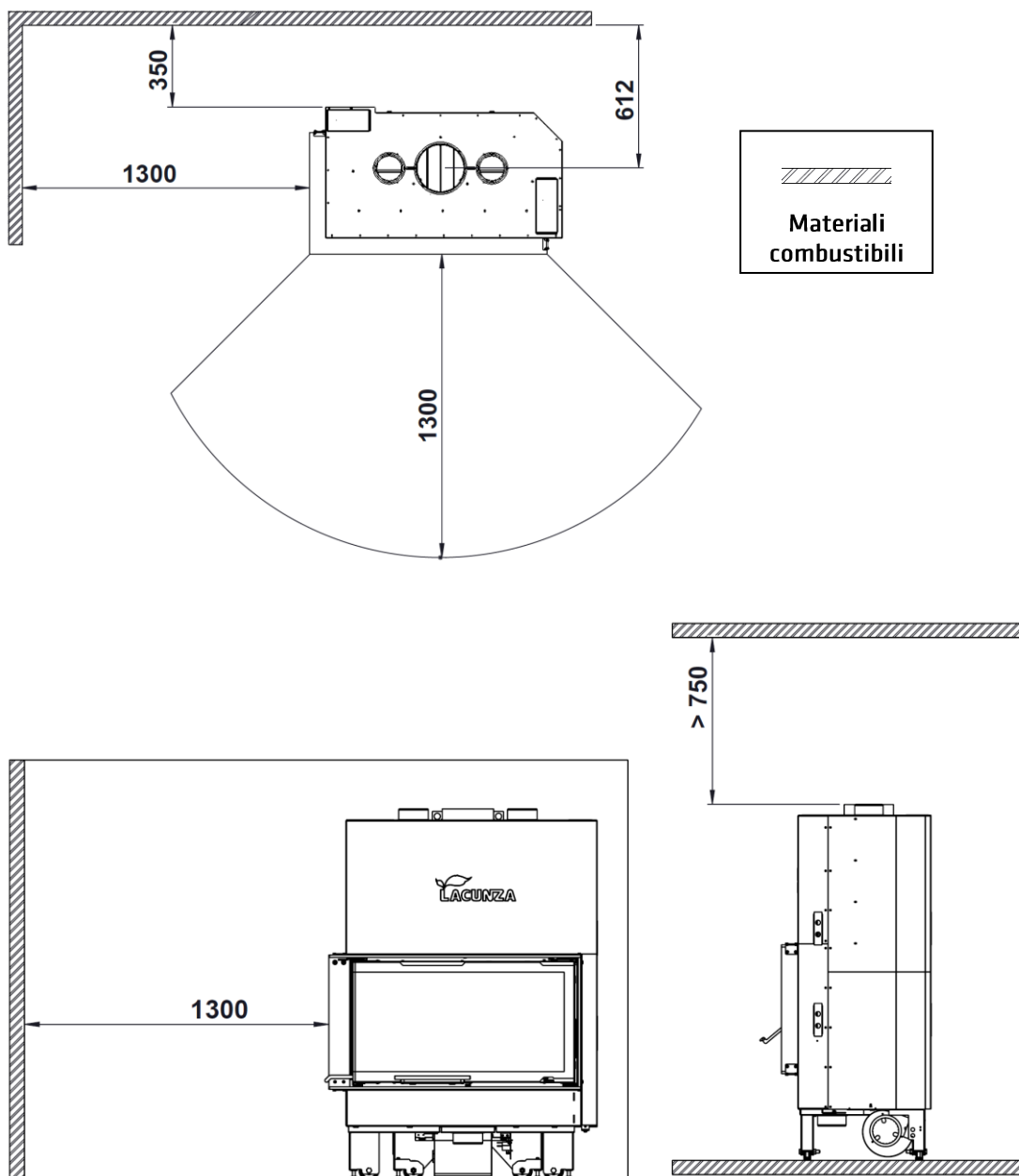
Figura n°5 - Distanze di sicurezza Izaro 80-100 CLI
