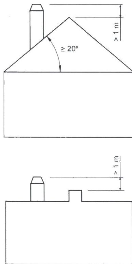
Figura n°23 - Distanza tra la finitura e il colmo del tetto
