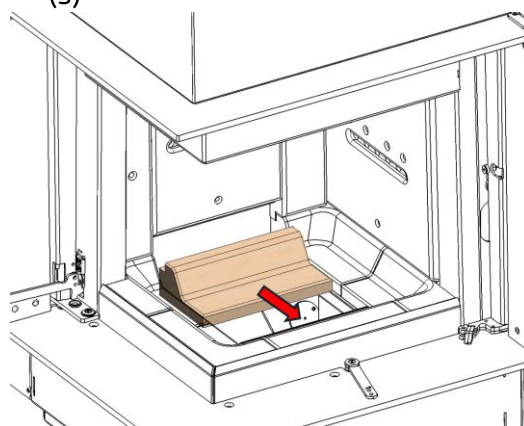
c- Rimuovere la base centrale posteriore (10) portandola in avanti
