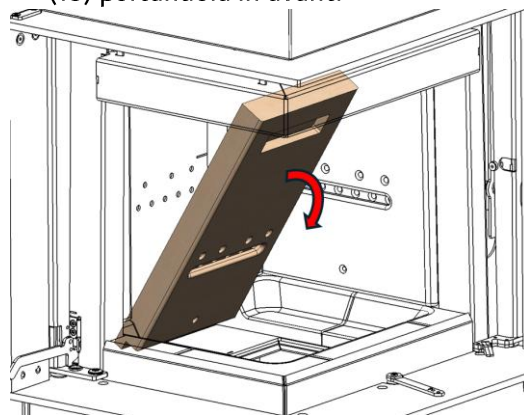
d- Rimuovere la piastra centrale posteriore (5) lasciandola cadere in avanti.
