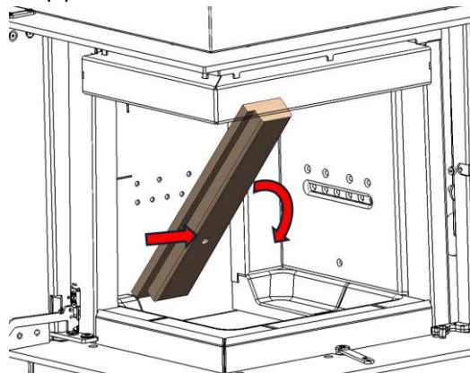
e- Rimuovere la piastra posteriore sinistra (4) spostandola verso l'interno e lasciandola cadere in avanti.
