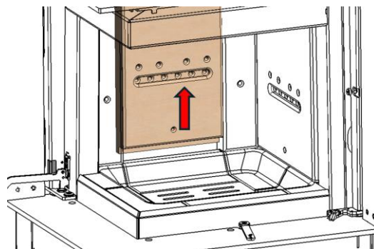
b- Sollevare la piastra posteriore centrale (5)
