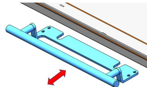
Figura n°45 - Estrazione delle viti e utilizzo come "maniglia fredda" per la maniglia
