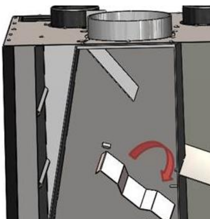
Figura n°33 - Smontaggio del deflettore intermedio Itaca 80
