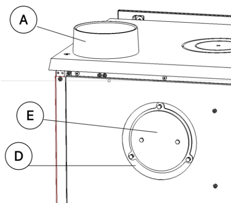
Figura n. 8 - Situazione finale, adatta per uscita fumi superiore.
