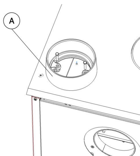
Figura n°6 - Posizioniamo la flangia superiore di uscita fumi.
