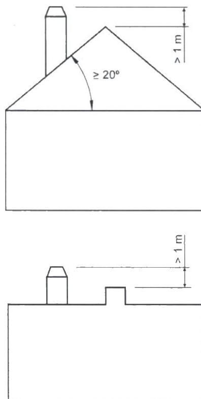
Figura n°8 - Distanza tra la finitura e il colmo del tetto
