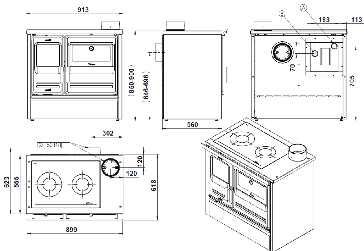
Figura n°2 - Dimensioni in mm dell'apparecchio Etna 7T E Extra V S. Sup Lat.
