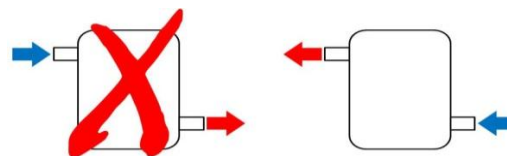
Figura n°11 - Collegamento scorretto (sin.) e collegamento corretto (dest.)
