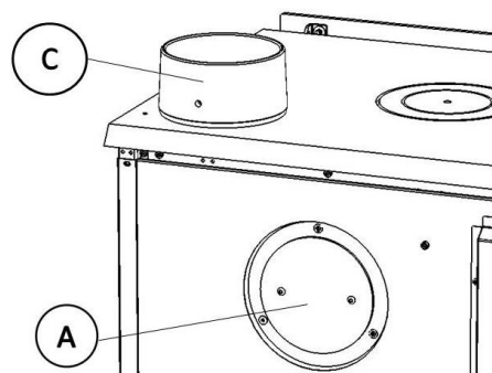
Figura n°9 - Schema per scarico fumi superiore
