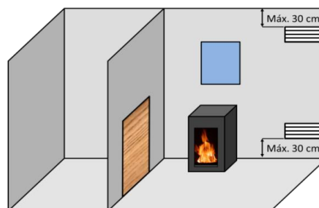
Figura n°5 - Schema orientativo per griglie di ventilazione
