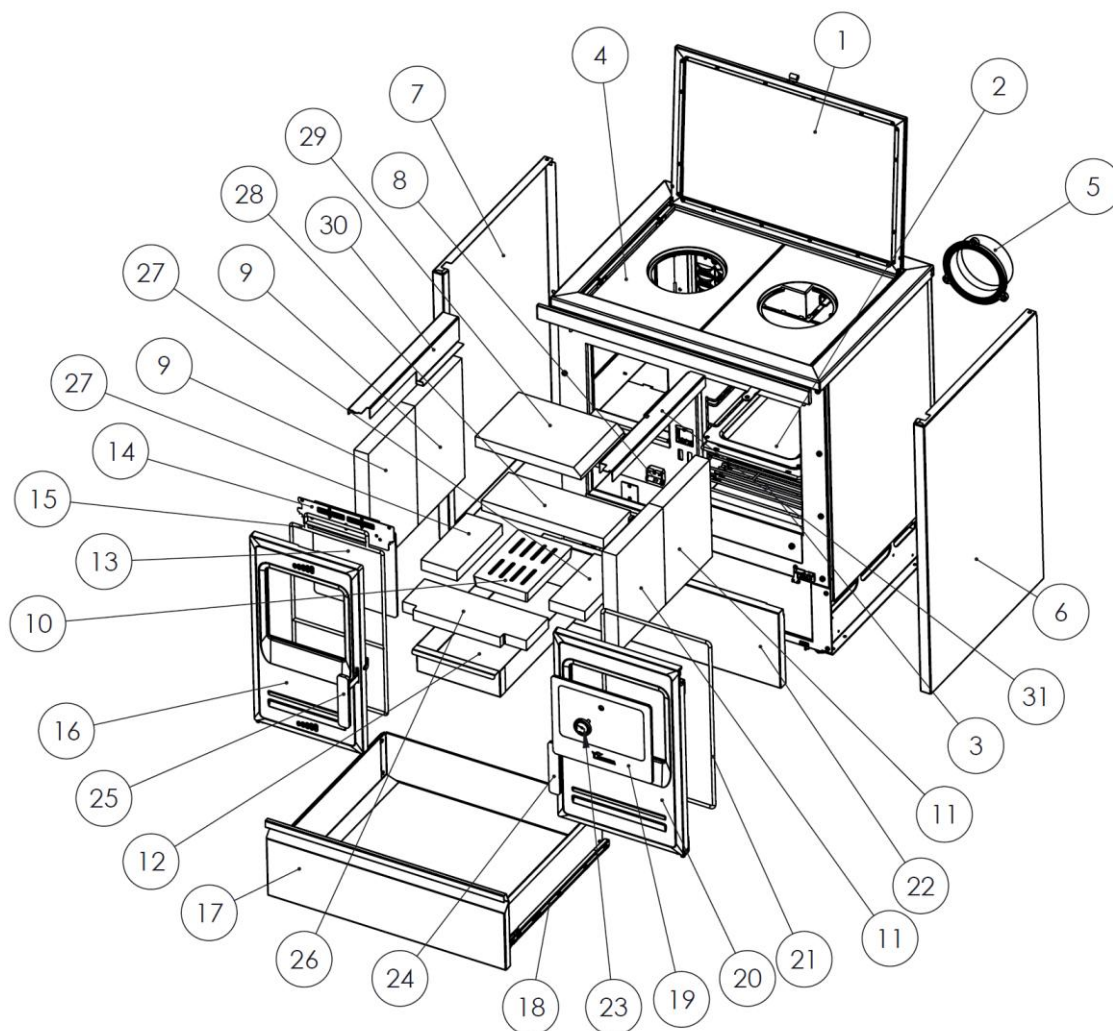
Figura nº26 - ETNA 5T
