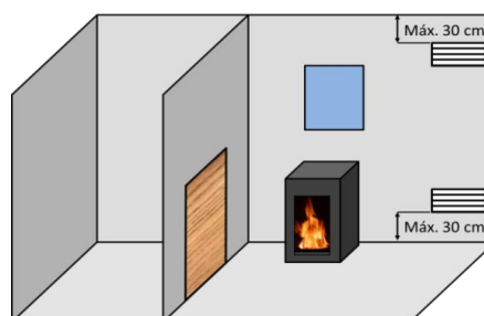
Figura n°7 - Schema orientativo per griglie di ventilazione
