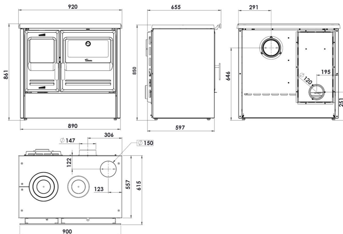
Figura n°5 - Dimensioni in mm dell'apparecchio ETNA 7T S-SUP
