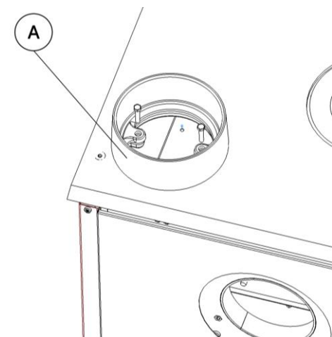
Figura n°10 - Posizioniamo la flangia superiore di uscita fumi.
