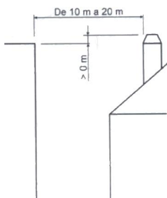
Figura nº16 - Distanza tra la finitura e oggetti tra 10 e 20 m
