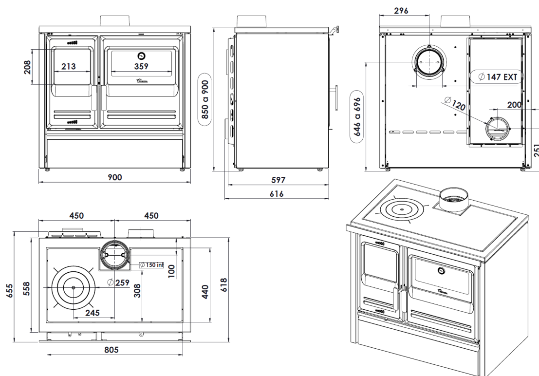
Figura n°6 - Dimensioni in mm dell'apparecchio ETNA 7T New
