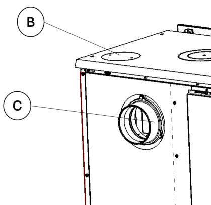
Figura n°9 - Situazione iniziale. Rilasciamo i pezzi indicati.
