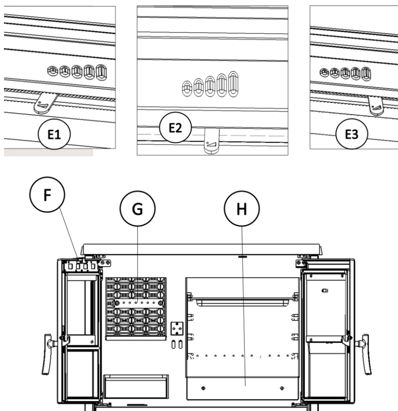
Figura n°18 - Elementi di funzionamento dell'apparecchio
