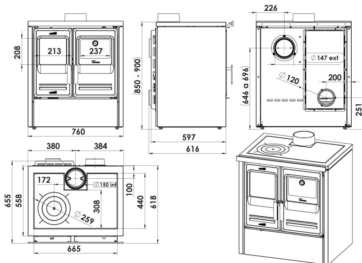
Figura n°3 - Dimensioni in mm dell'apparecchio ETNA 5T New
