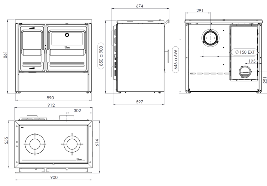
Figura n°4 - Dimensioni in mm dell'apparecchio ETNA 7T TOP
