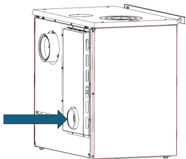
Figura n°13 - Condotto dell'aria per la camera di combustione.
