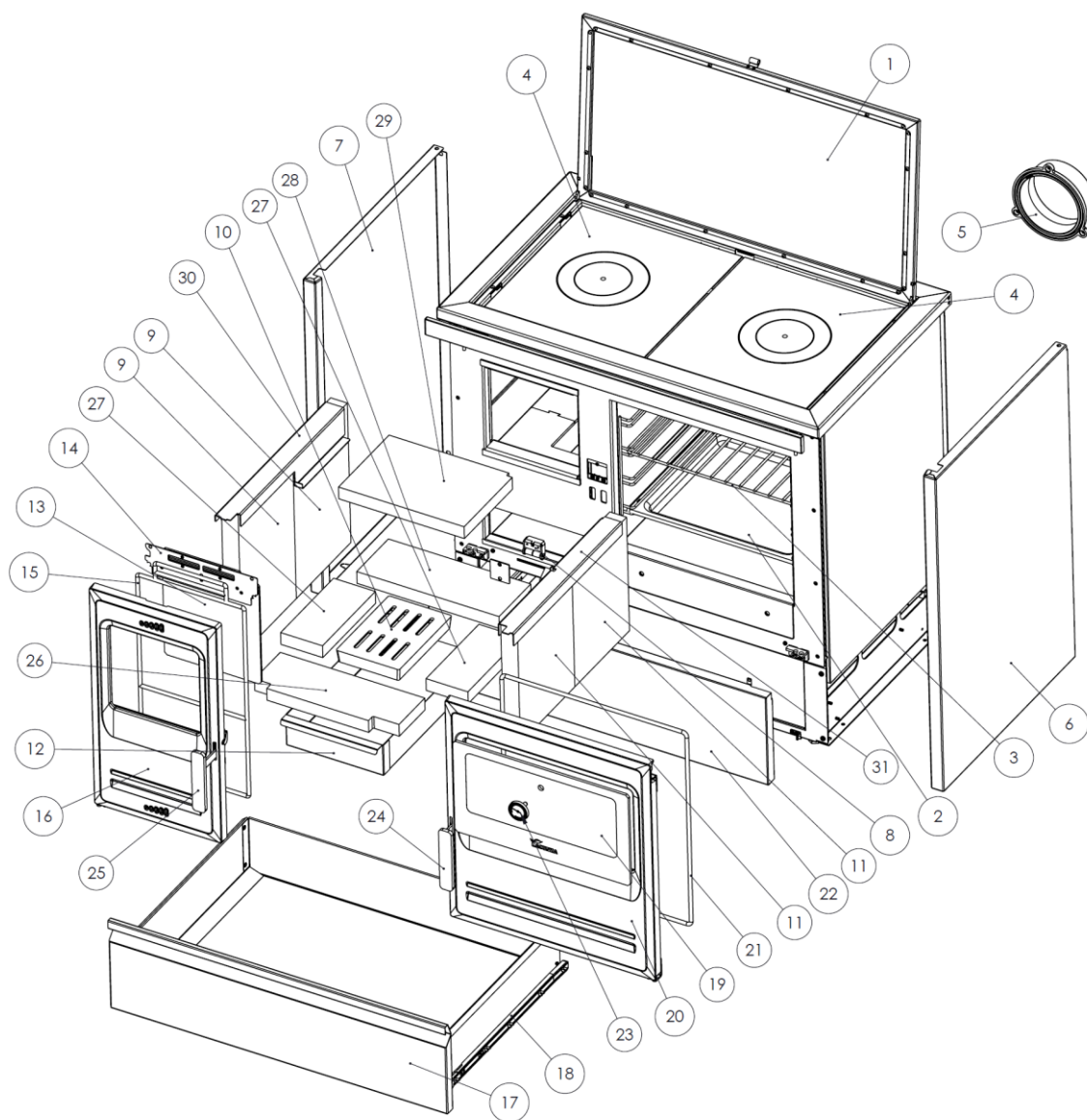
Figura nº27 - ETNA 7T
