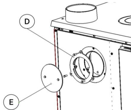
Figura n°11 - Posizioniamo l'adattatore e il coperchio
