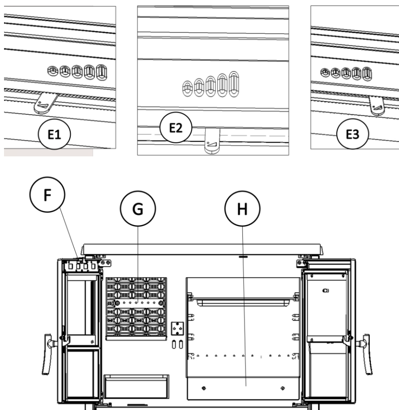
Figura n°16 - Elementi di funzionamento dell'apparecchio
