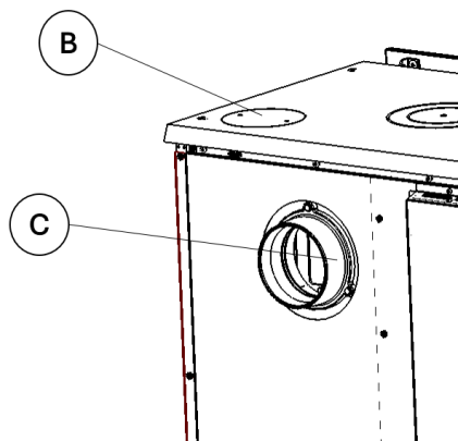
Figura n°7 - Situazione iniziale. Rilasciamo i pezzi indicati.
