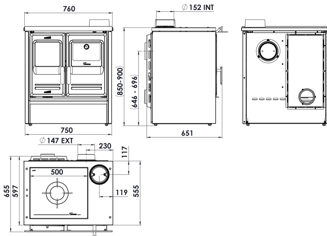
Figura n°1 - Dimensioni in mm dell'apparecchio ETNA 5T E/V S-SUP
