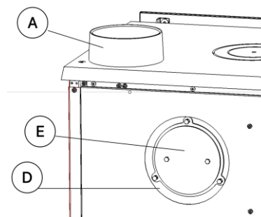
Figura n°10 - Figura n. 8 - Situazione finale, adatta per uscita fumi superiore.
