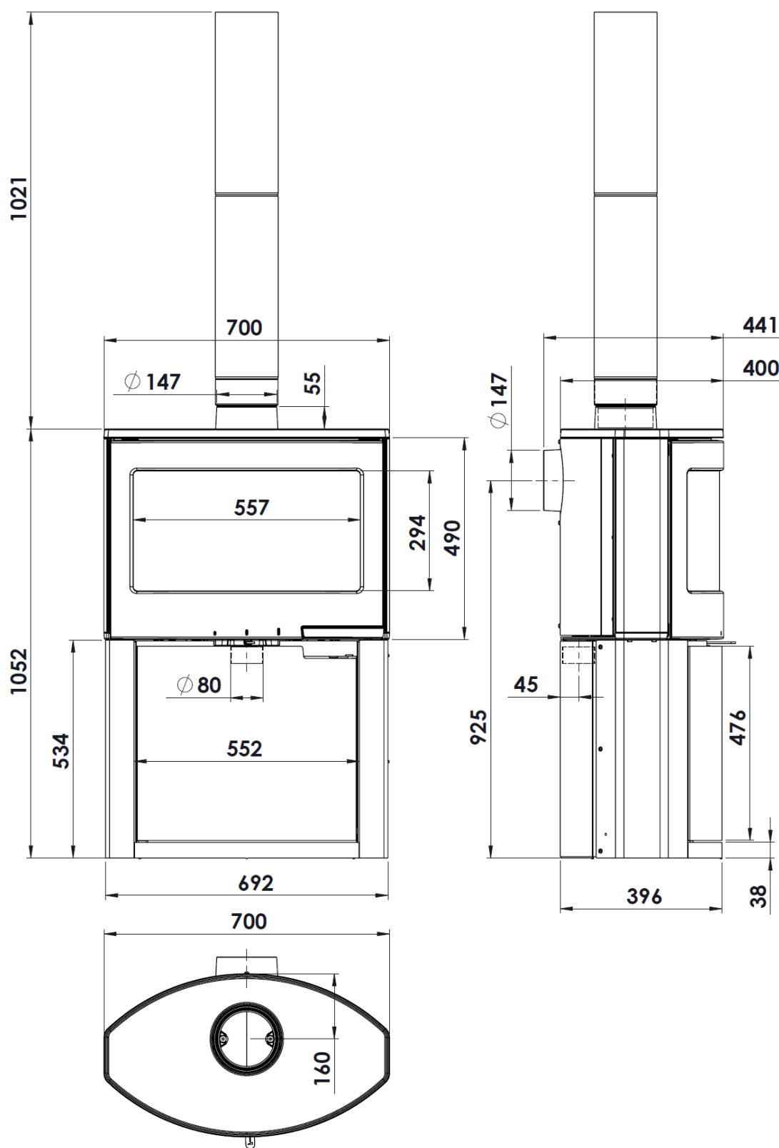
Figura n°2 - Dimensioni in mm dell'apparecchio Bera Star
