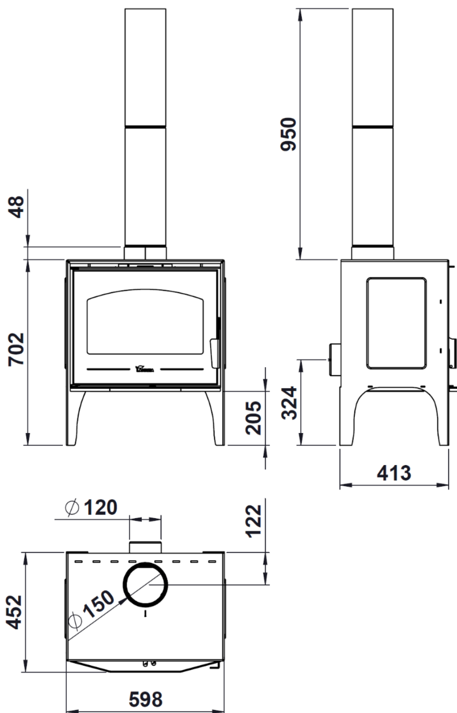
Figura n°1 - Dimensioni in mm dell'apparecchio serie CALPE STAR
