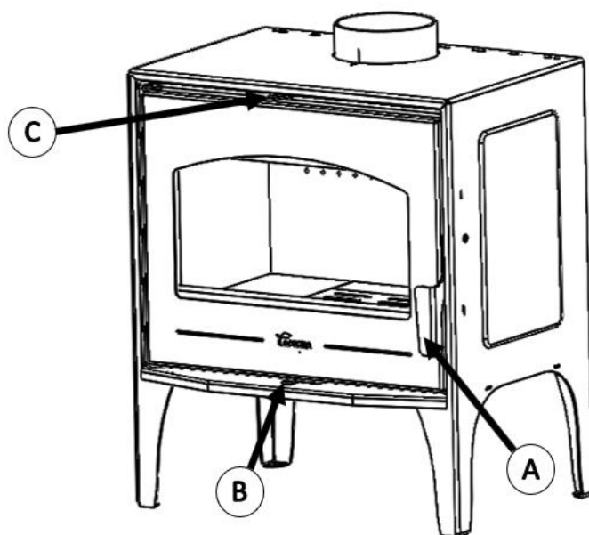
Figura n°8 - Elementi di funzionamento dell'apparecchio
