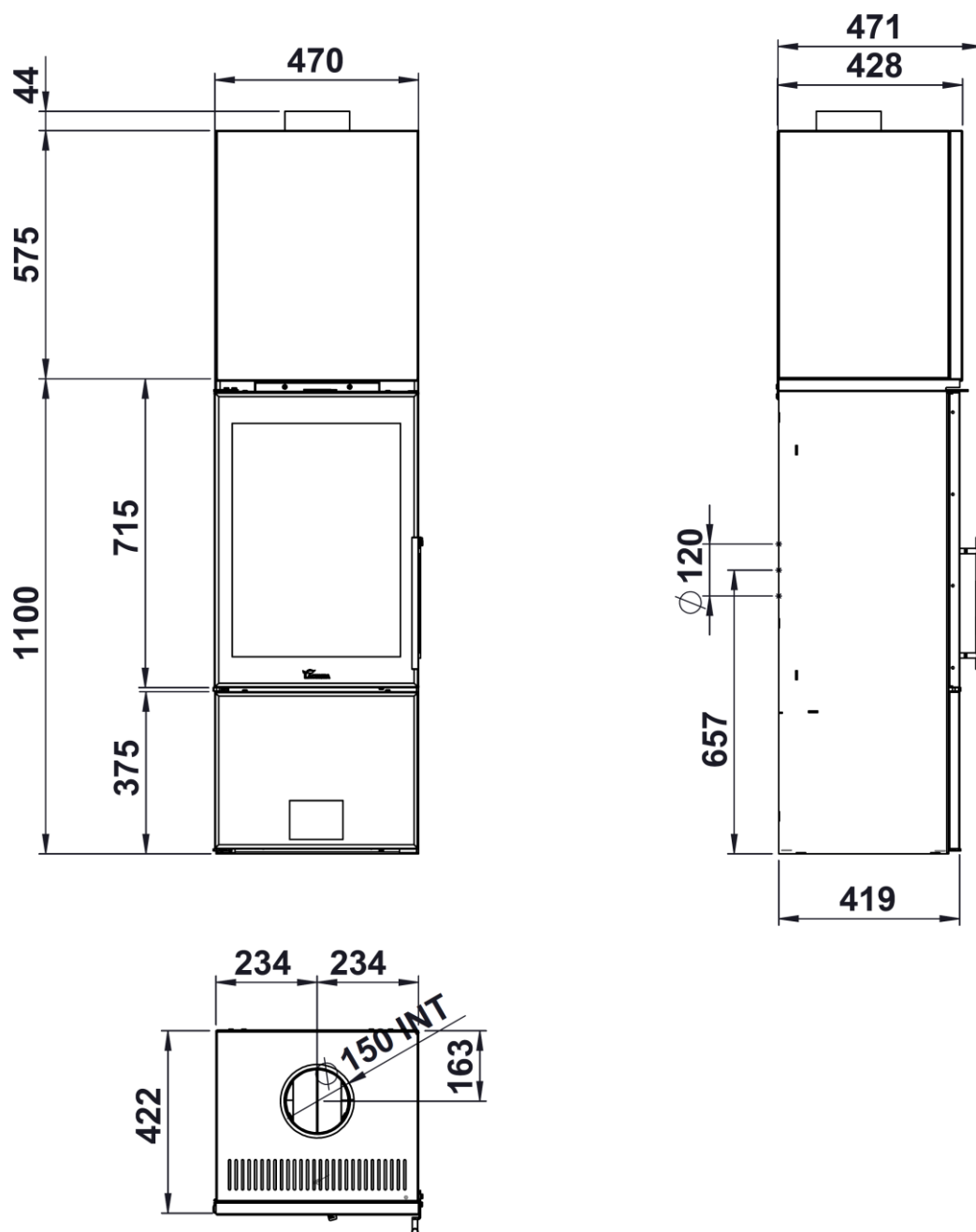
Figura n°1 - Dimensioni in mm dell'apparecchio serie Calais +EX151
