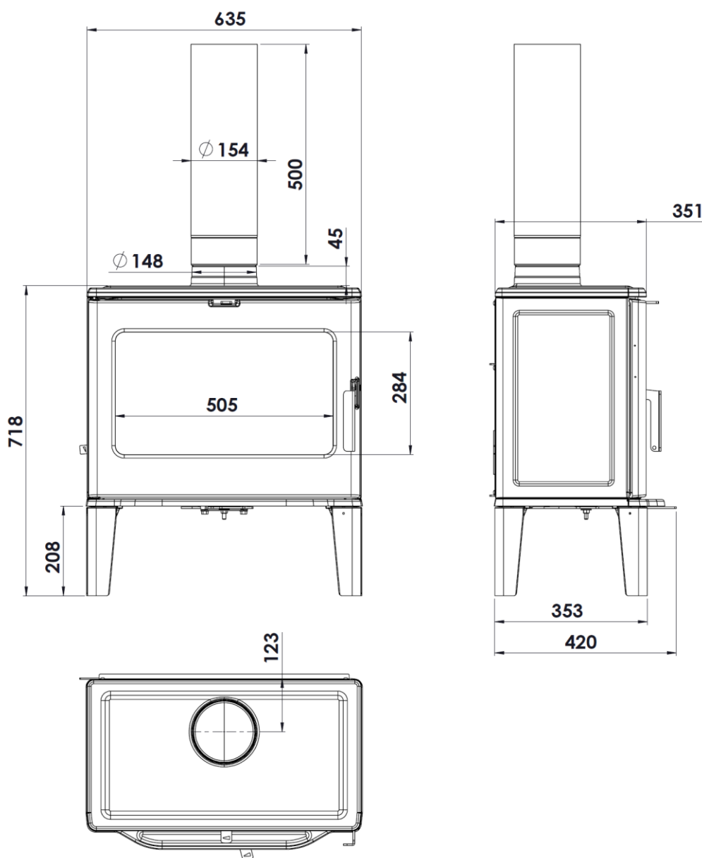
Figura n°1 - Dimensioni in mm dell'apparecchio Bidart
