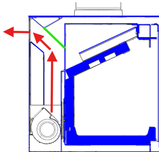
Figura n°13 - Percorso dell'aria calda con canalizzazione
