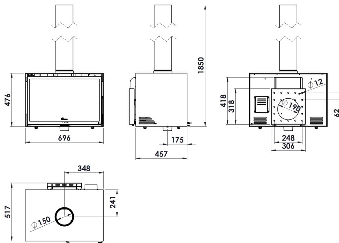
Figura n°2 - Dimensioni in mm dell'apparecchio BAIONA 700 STAR MURAL
