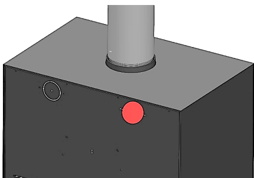
Figura n°7 - Rimuovere la lamiera circolare
