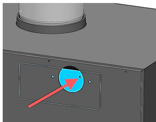
Figura n°9 - Cambiare la posizione della lamiera interna spingendola verso l'interno.
