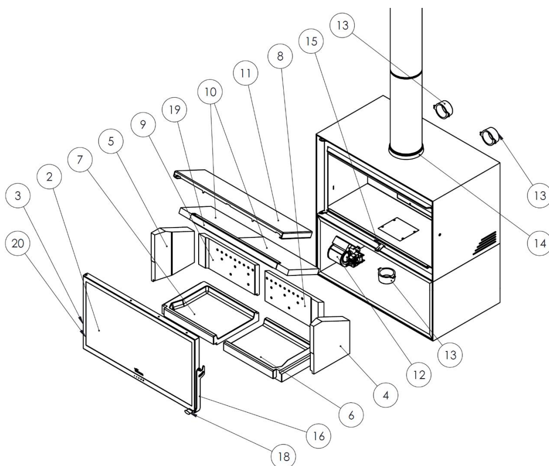
Figura n°24 - Baiona 700-800 Star
