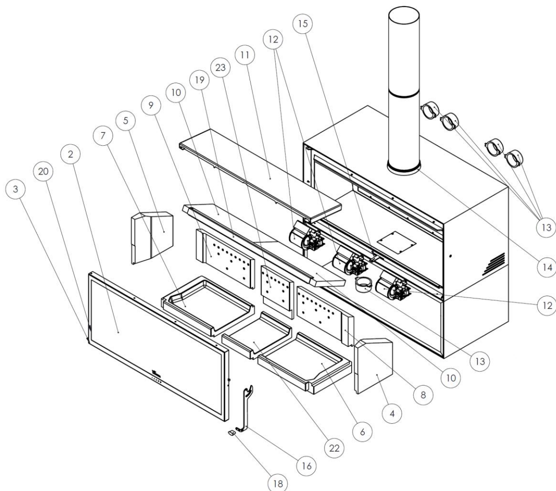
Figura nº25 - Baiona 1000 Star
