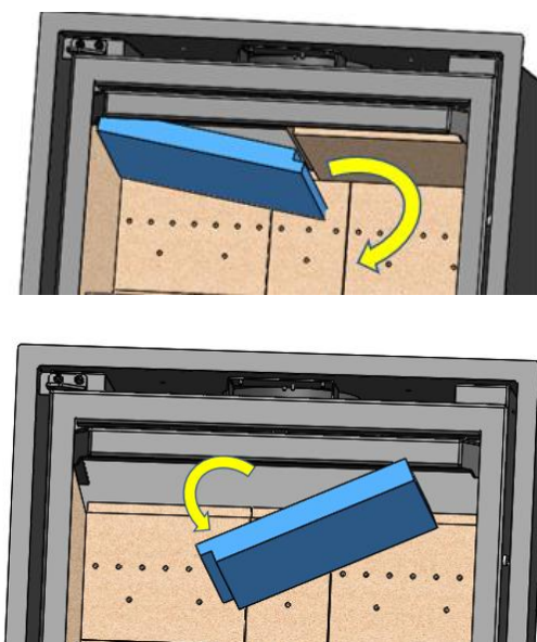
Figura n°21 - Smontaggio di deflettori inferiori
