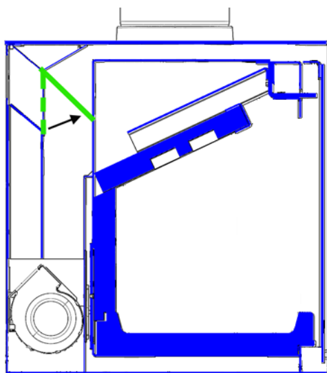
Figura n°12 - Spingere la lamiera interna fino all'arresto
