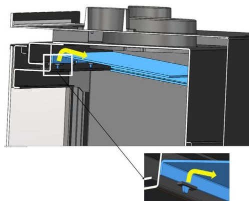
Figura n°22 - Smontaggio del deflettore superiore in acciaio
