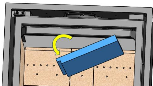
Figura n°23 - Smontaggio di deflettori inferiori
