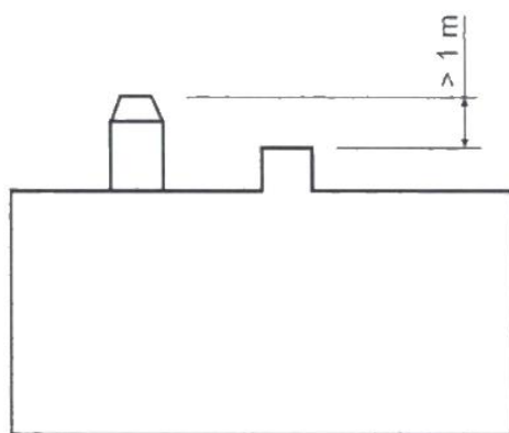
Figura nº14 - Distâncias desde o acabamento até à cumeeira do telhado
