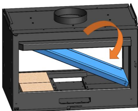
Figura nº23 - Solte o defletor e retire-o da fôrma
